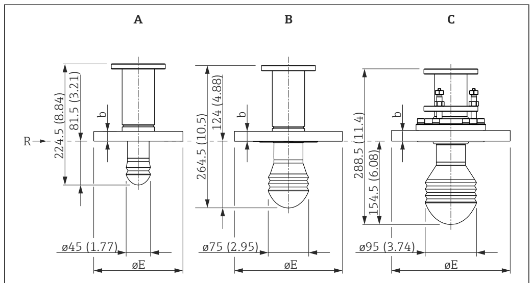
12 Wymiary anten; jednostka miary: mm (cale)
