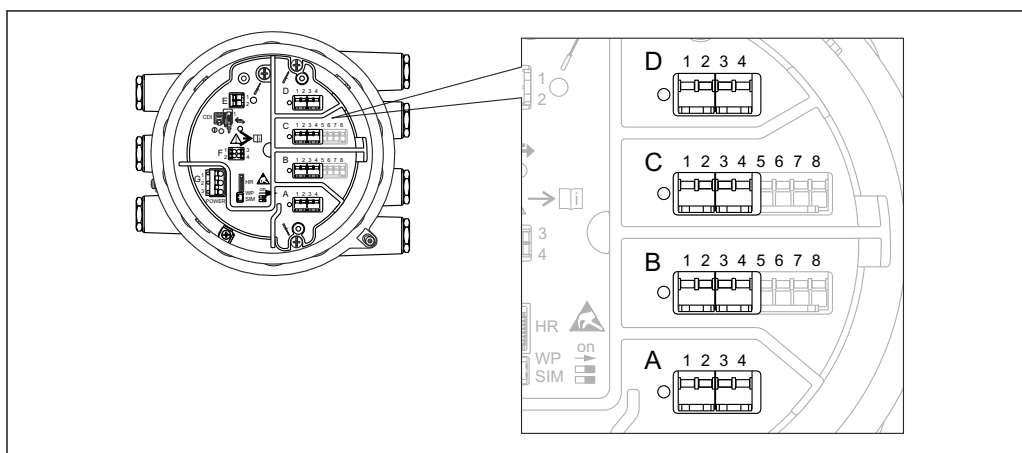
6 Położenie dodatkowych portów I/O w przedziale podłączeniowym
