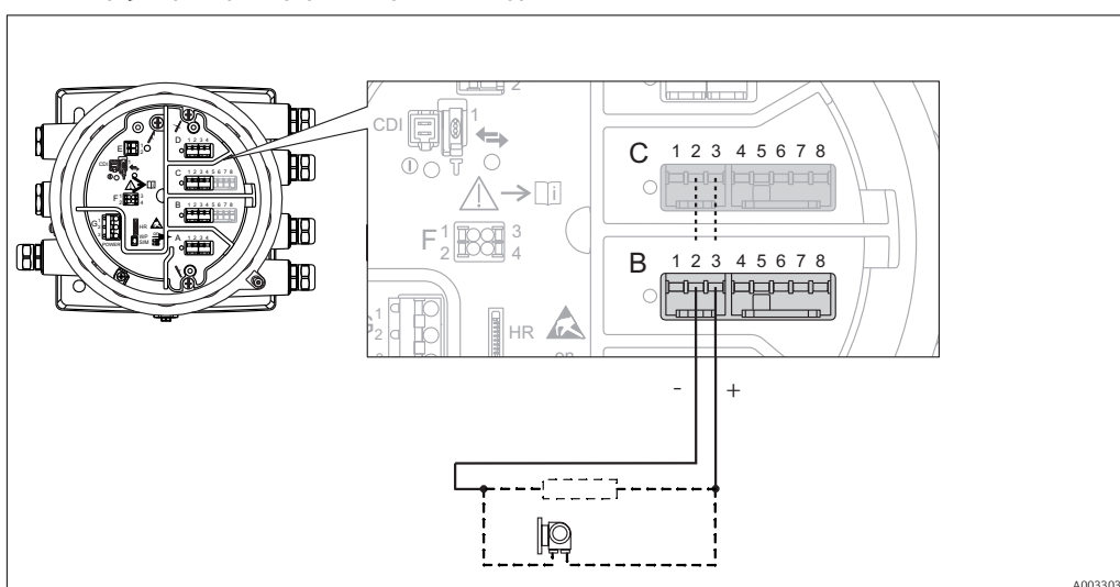
8 Wejście lub wyjście aktywne: użyć zacisków 2 i 3
