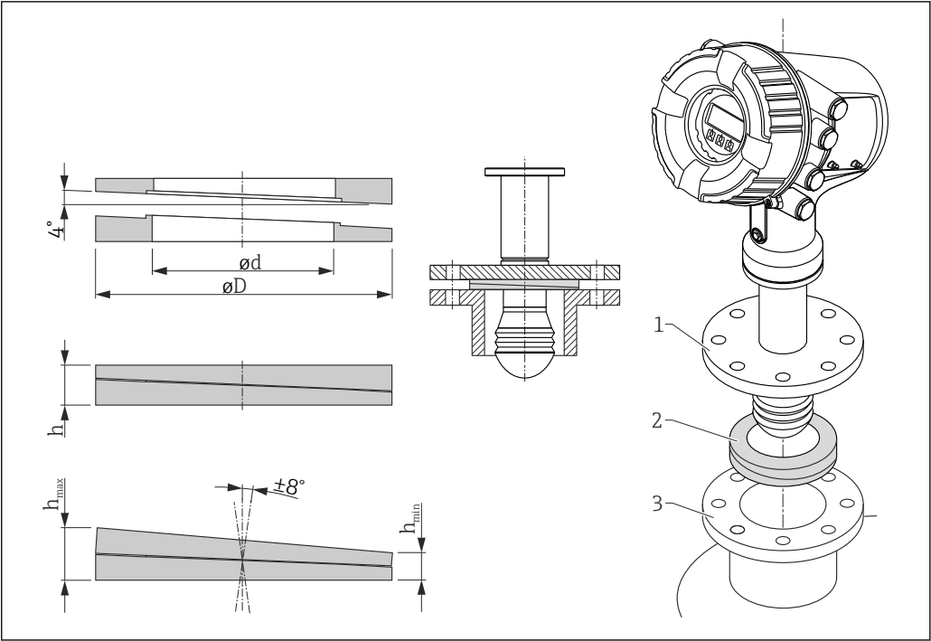
19 Kołnierz pozycjonujący umożliwia regulację pozycji anteny po kątem \pm 8^\circ
