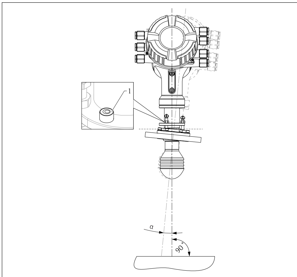
10 Pozycjoner anten o średnicy 100 mm (4")
