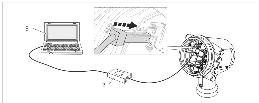
16 Obsługa poprzez interfejs serwisowy
