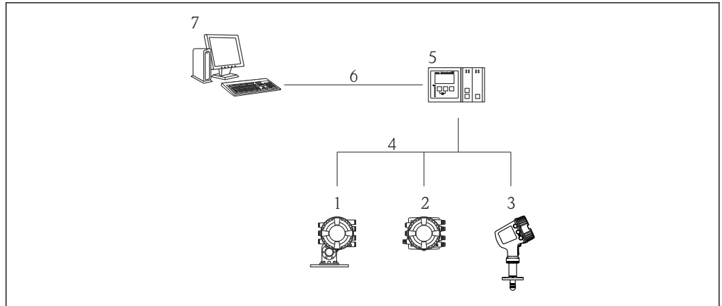
15 Obsługa zdalna przyrządów do pomiarów zawartości zbiorników
