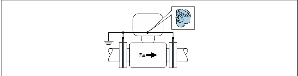
3 Potenzialausgleich über Erdungsklemme und Erdungsscheiben
