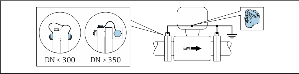
4 通过接地端子和管道法兰实现电势平衡
