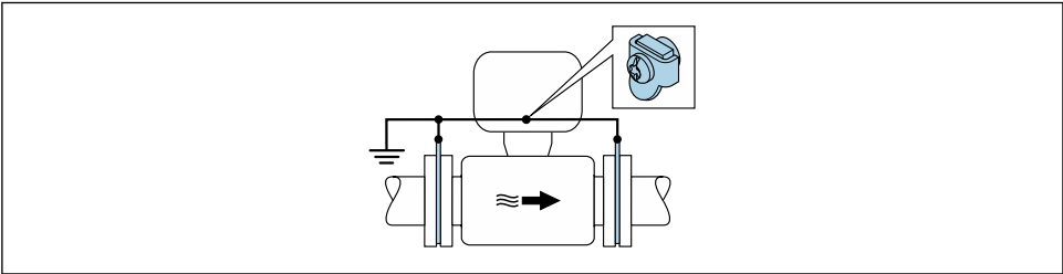
5 通过接地端子和接地环实现系统电势平衡
