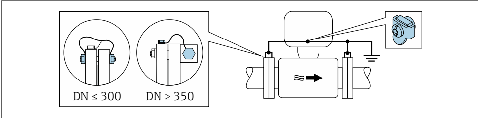
図 3 接地端子および配管フランジを介した電位平衡
