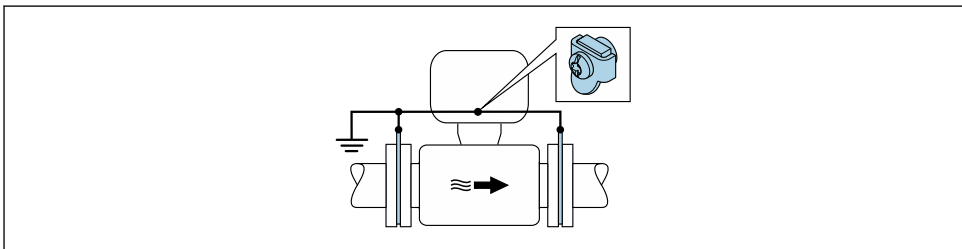
図 4 接地端子およびアースリングを介した電位平衡
