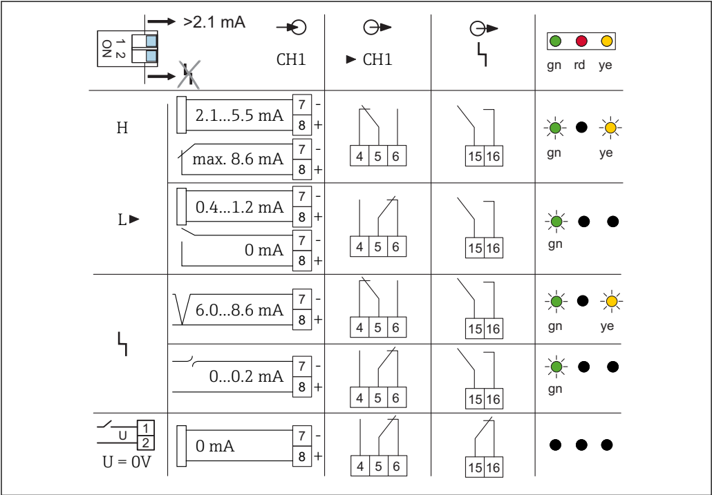
18 Sinal de limite L sem sinalização de falha (FEL58, FEL48, FEL68, FEM58, FEI58)
