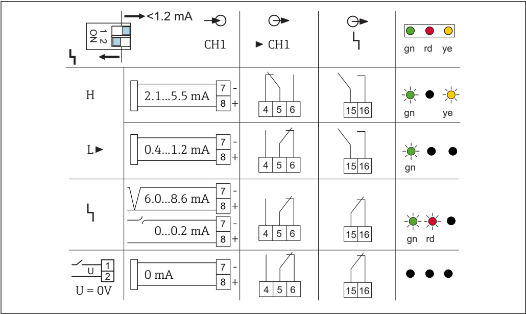
17 Sinal do limite L com sinalização da falha (FEL58, FEL48, FEL68, FEM58, FEI58)
