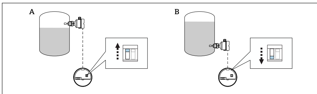
14 Posição da seletora na unidade eletrônica
