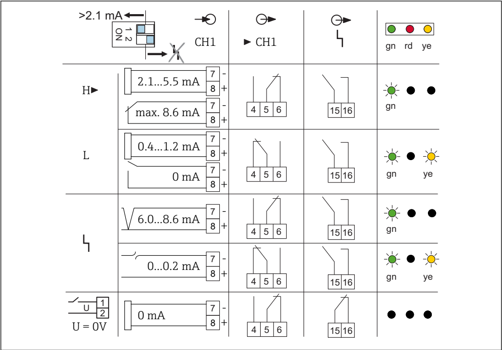
16 Sinal de limite H sem sinalização de falha (FEL56)
