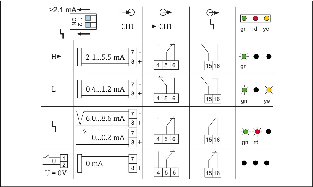
15 Sinal do limite H com sinalização da falha (FEL56)
