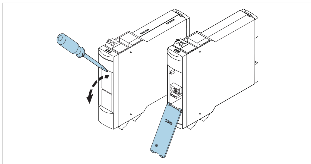
图 10 打开前面板
