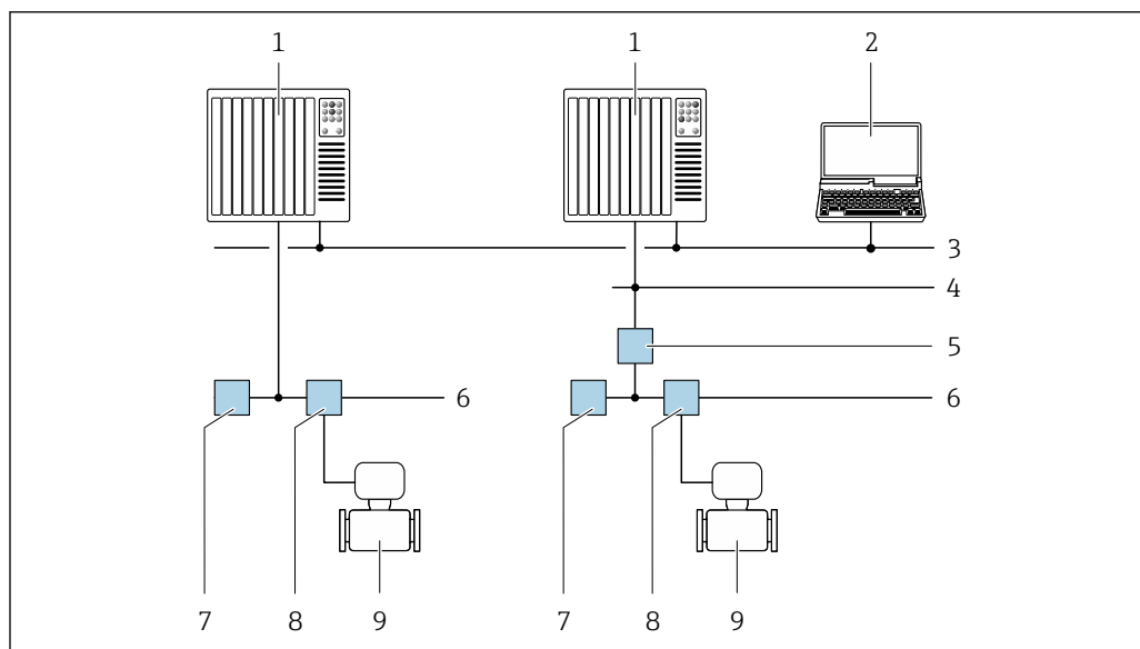
図 42 FOUNDATION フィールドバスネットワークを介したリモート操作のオプション
