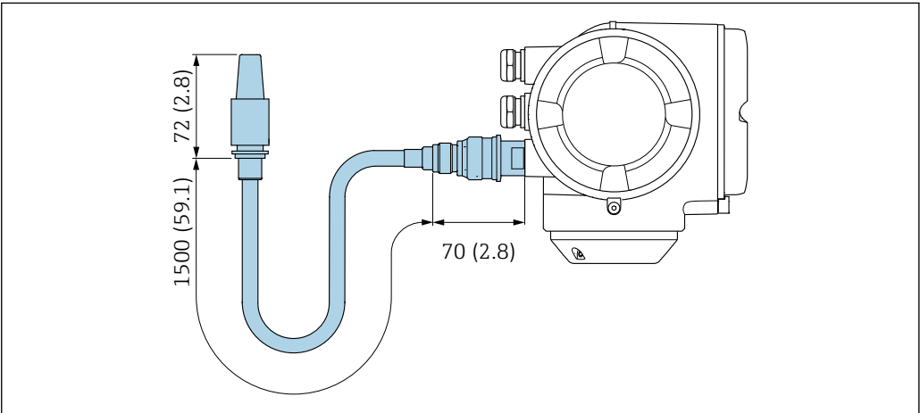
33 単位 mm (in)
