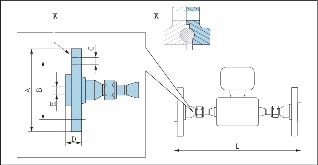
図 30 X の詳細：非対称型プロセス接続；着色部分が供給されます。
