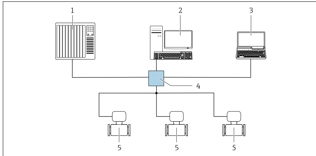
図 45 EtherNet/IP ネットワーク経由のリモート操作オプション：スター型トポロジー
