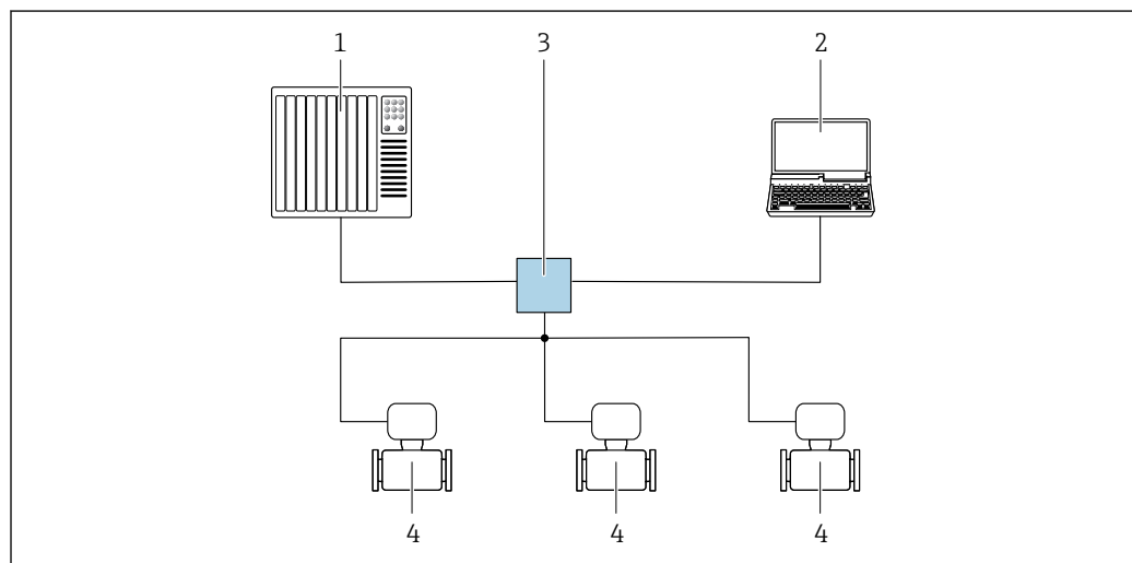
図 47 PROFINET ネットワーク経由のリモート操作オプション：スター型トポロジー
