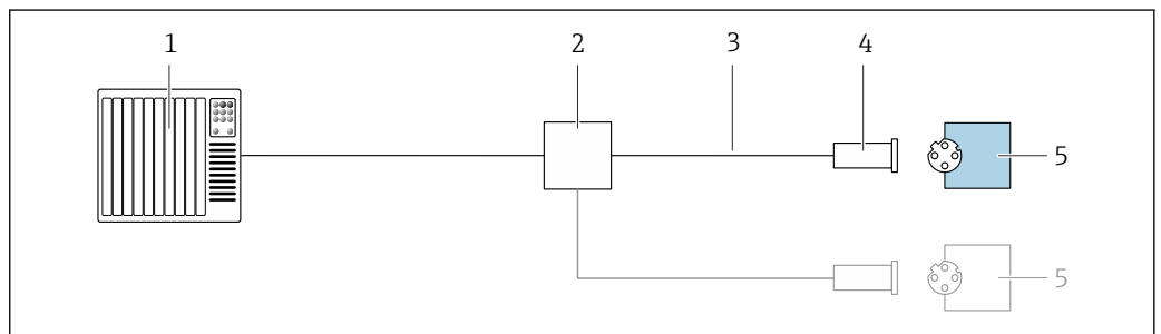
図 7 PROFINET の接続例
