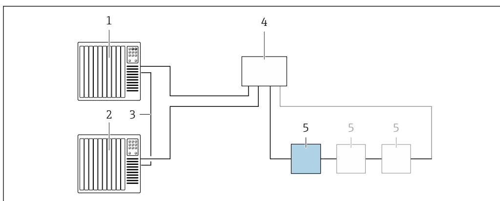
図 8 システム冗長 S2 の接続例
