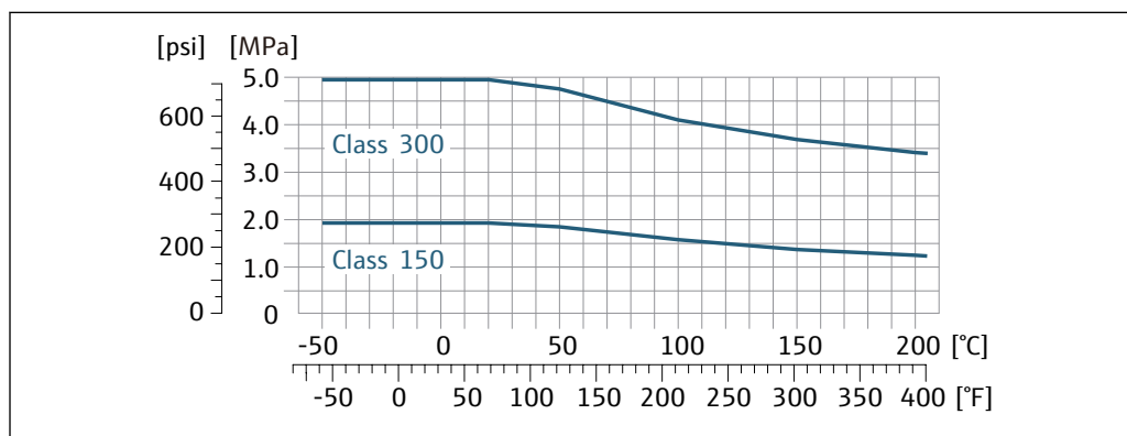
図 24 フランジ材質：1.4539 (SUS 890L 相当)、アロイ C22；ラップジョイントフランジ（非接液）：1.4404 (SUS F316L 相当)
