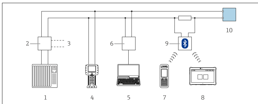
図 41 HART プロトコル経由のリモート操作用オプション（パッシブ）
