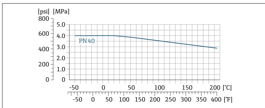
図 23 フランジ材質：1.4539 (SUS 890L 相当)、アロイ C22；ラップジョイントフランジ（非接液）：1.4404 (SUS F316L 相当)
