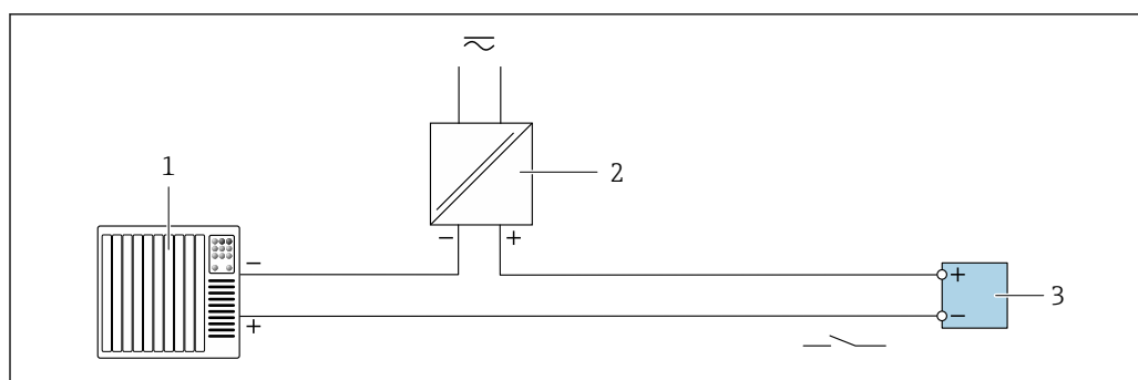
図 17 リレー出力（パッシブ）の接続例
