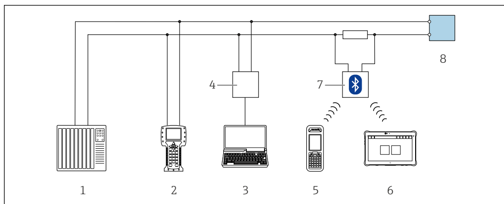
図 40 HART プロトコル経由のリモート操作用オプション（アクティブ）
