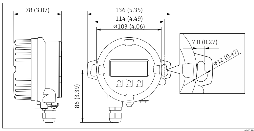
図 34 単位 mm (in)
