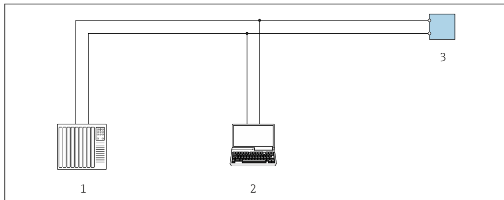
図 44 Modbus-RS485 プロトコル経由のリモート操作オプション（アクティブ）
