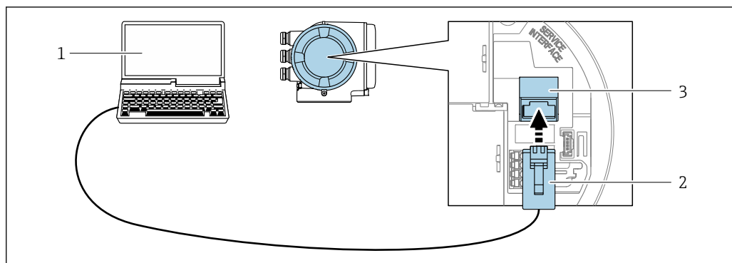
図 49 サービスインターフェイス（CDI-RJ45）経由の接続
