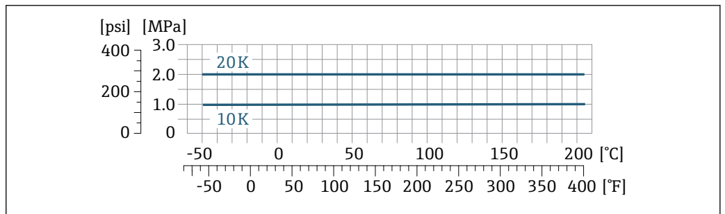
25 フランジ材質：1.4539 (SUS 890L 相当)、アロイ C22；ラップジョイントフランジ（非接液）：1.4404 (SUS F316L 相当)
