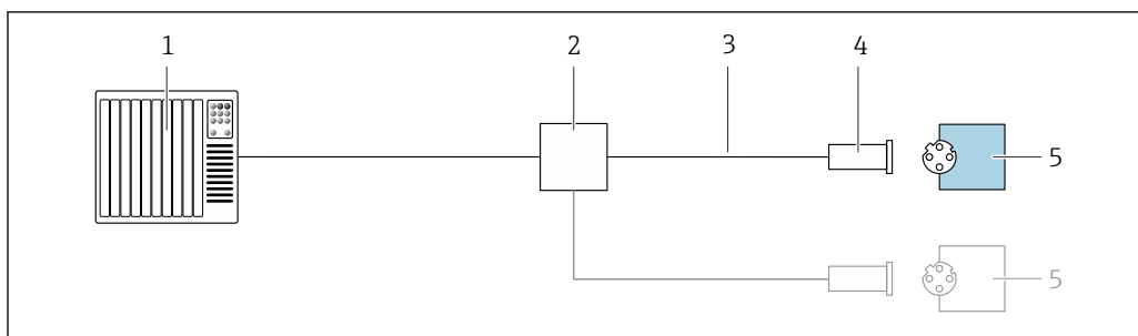
6 Пример подключения для EtherNet/IP
