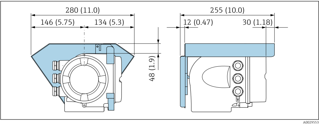
27 Защитный козырек от погодных явлений для Proline 500
