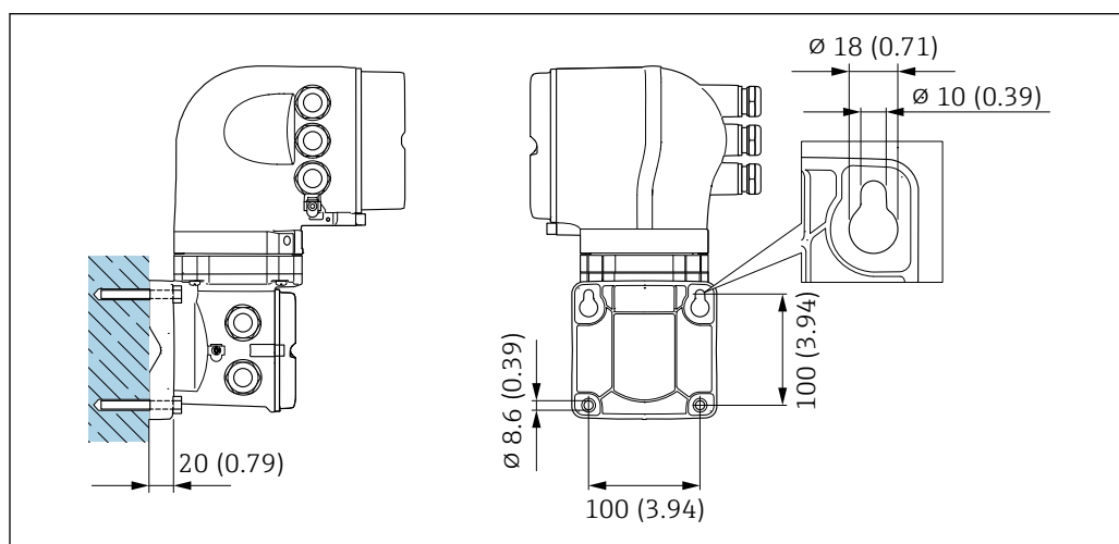
24 Единица измерения, мм (дюйм)
