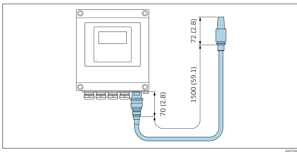
46 Единица измерения, мм (дюйм)
