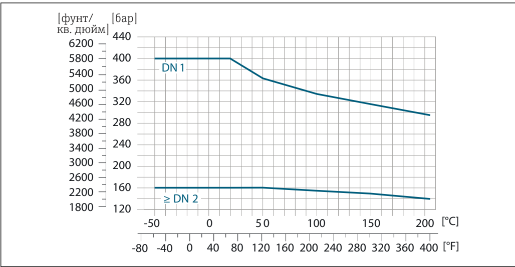
33 С фланцевым соединением 4-VCO-4: сплав Alloy C22. Переходник с резьбой ¼ NPTF: сплав Alloy C22. Соединение SWAGELOK ¼" или ½": 1.4401 (316L)
