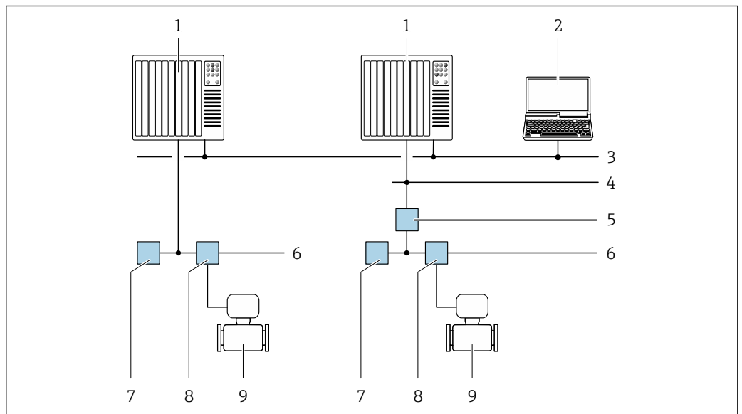
53 Варианты дистанционного управления через сеть FOUNDATION Fieldbus
