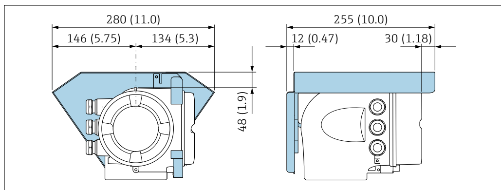
38 Защитный козырек от погодных явлений для Proline 500
