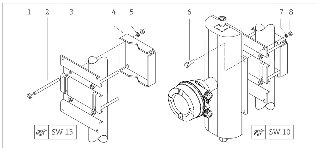
25 Комплект держателя для монтажа на опоре
