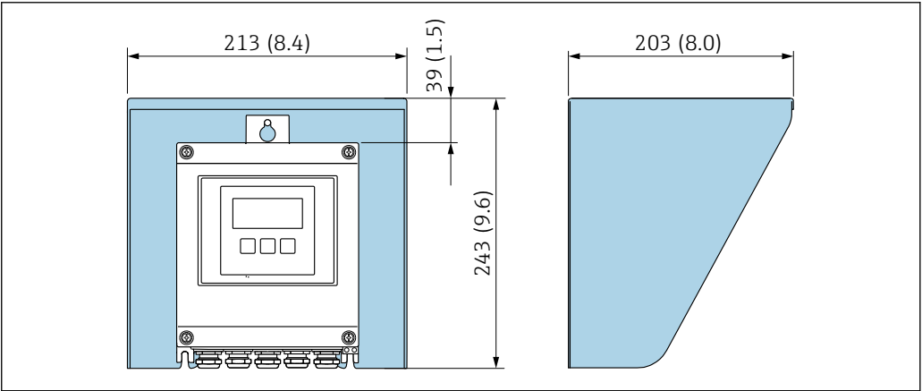
43 Защитный козырек от погодных явлений для Proline 500 – цифровое исполнение
