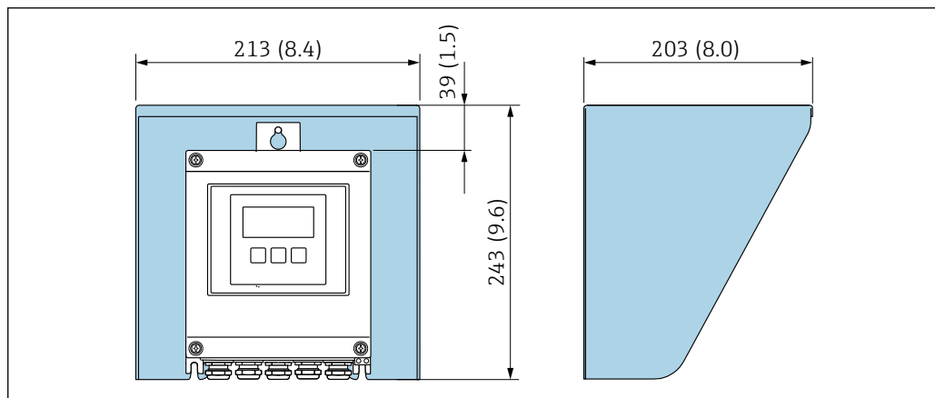
37 Защитный козырек от погодных явлений для Proline 500 – цифровое исполнение
