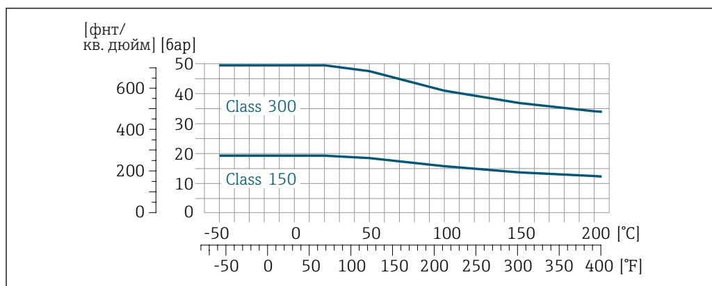
30 С фланцем из материала 1.4539 (904L), сплав Alloy C22; поворотные (не смачиваемые) фланцы из материала 1.4404 (SUS F316L)
