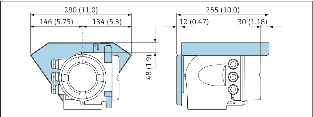
44 Защитный козырек от погодных явлений для Proline 500
