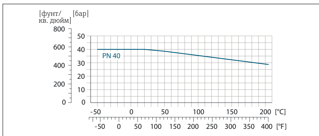
29 С фланцем из материала 1.4539 (904L), сплав Alloy C22; поворотные (не смачиваемые) фланцы из материала 1.4404 (SUS F316L)
