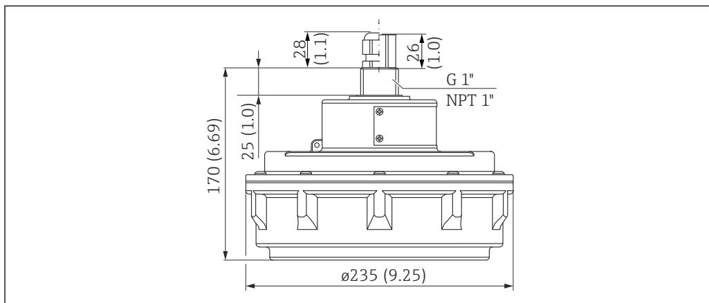
図 8 寸法。測定単位 mm (in)
