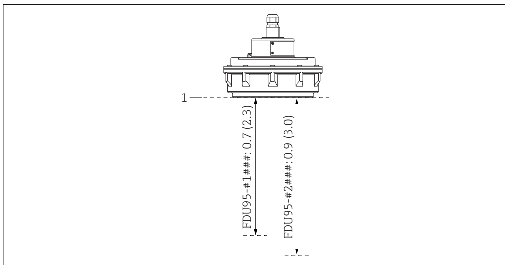
図 1 超音波センサの不感帯：単位 m (ft)
