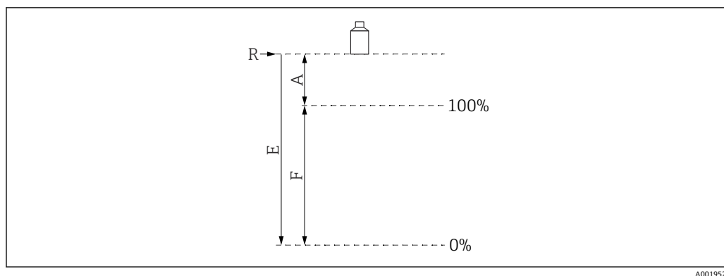
図 10 スパンを定義するための変数
