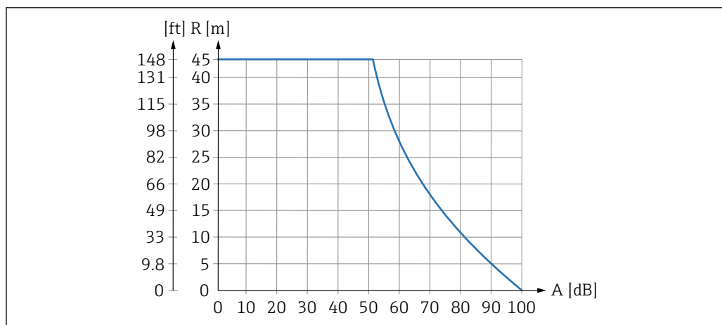
図 2 超音波センサの範囲グラフ
