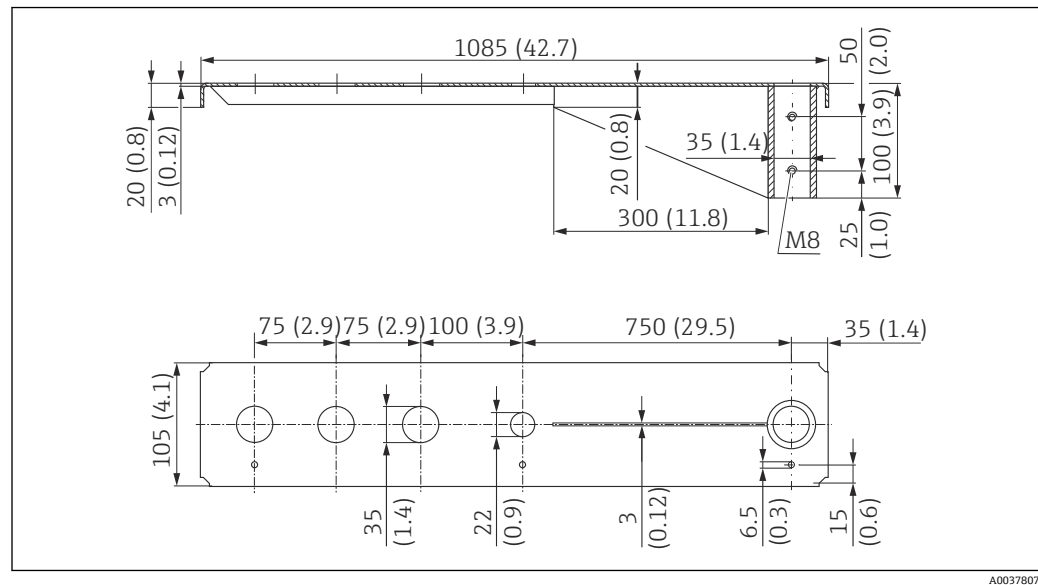
図 18 寸法。測定単位 mm (in)
