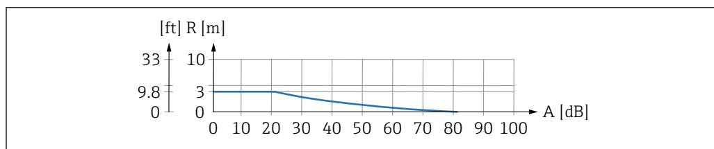
図 2 超音波センサの範囲グラフ
