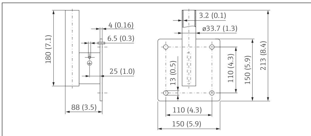
図 21 壁面ブラケットの寸法。測定単位 mm (in)
