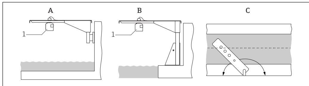
図 7 開水路またはフリーム上のカンチレバーアームを使用した設置
