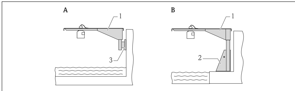
■ 16 カンチレバーアームを使用したセンサの取付け
