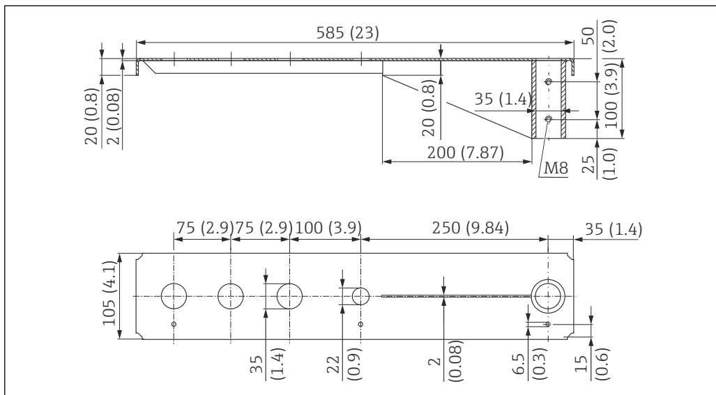
■ 17 寸法。測定単位 mm (in)
