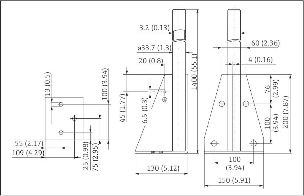
20 寸法。測定単位 mm (in)
