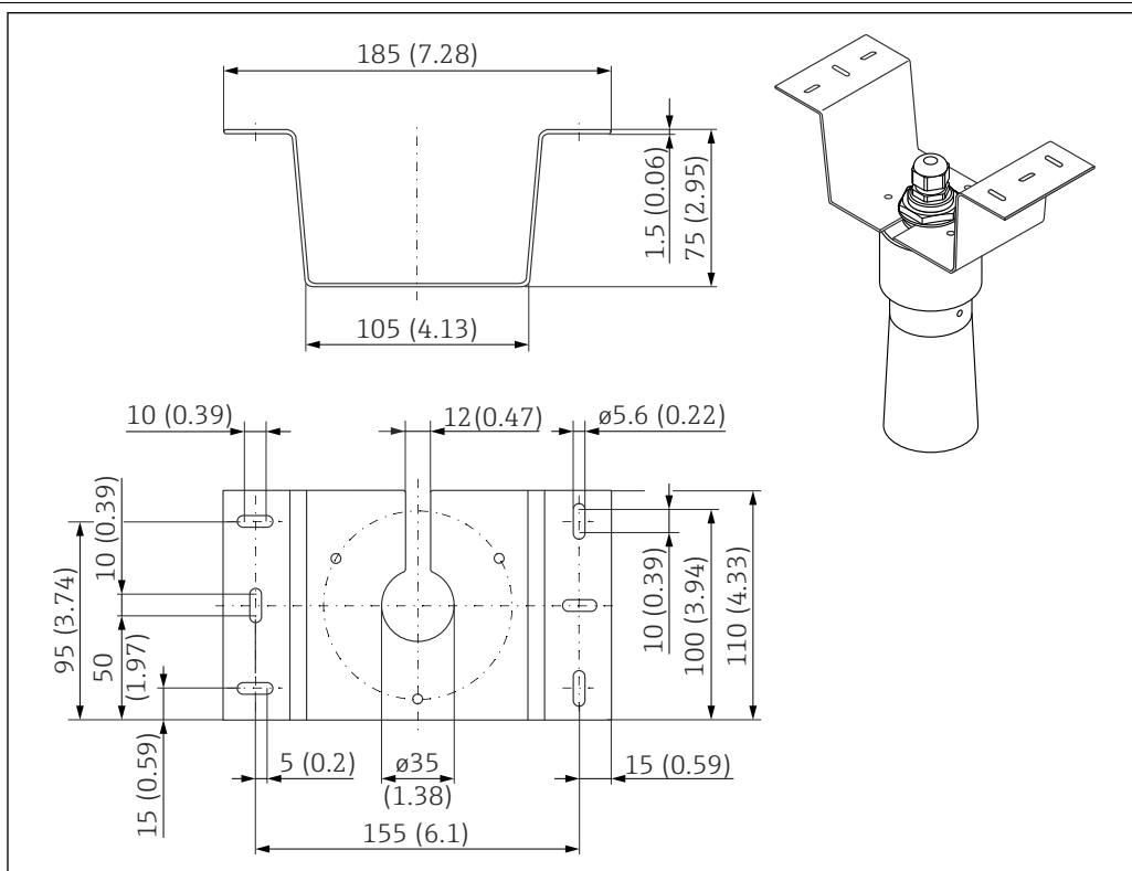
図 22 天井取付け用の取付ブラケット。測定単位 mm (in)
