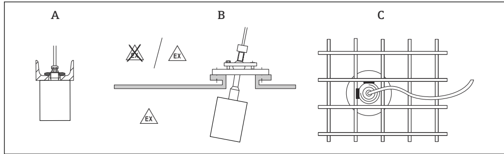
図 6 システム内に設置
