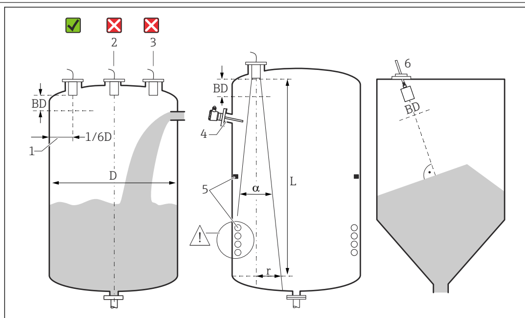
図 5 レベル計の設置条件
