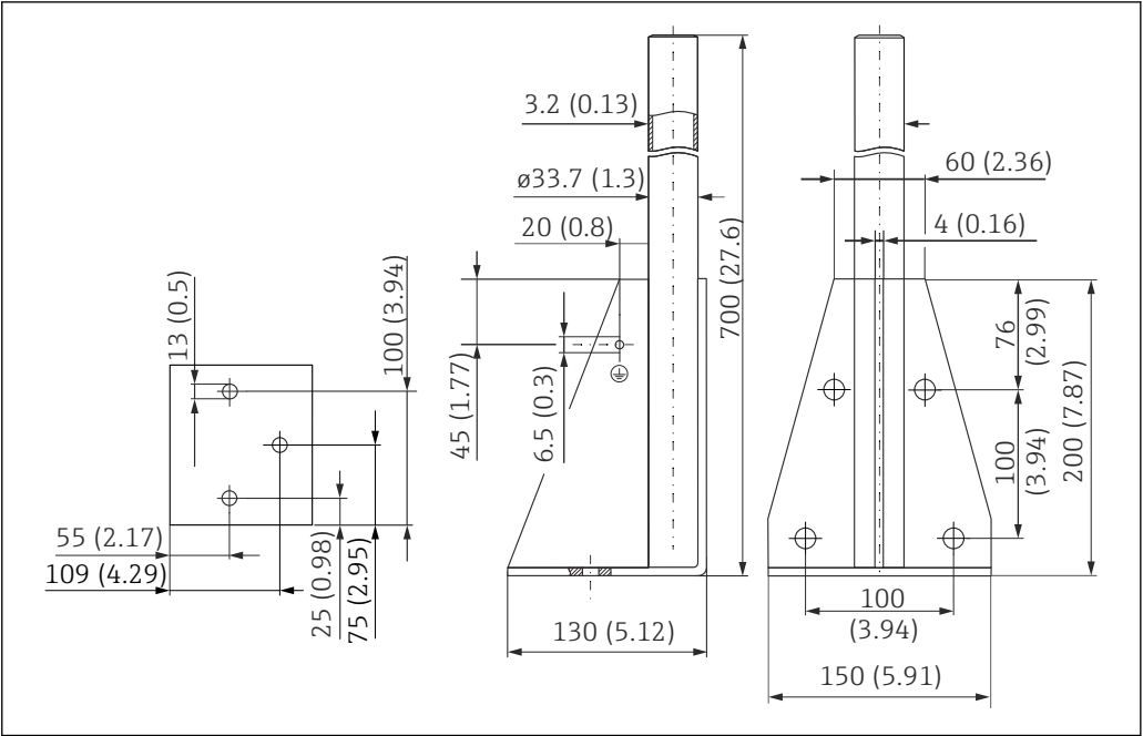
19 寸法。測定単位 mm (in)
