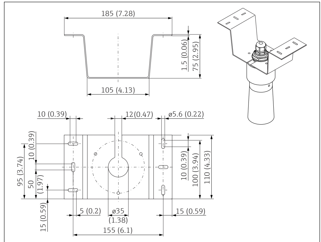
20 天井取付け用の取付ブラケット。測定単位 mm (in)
