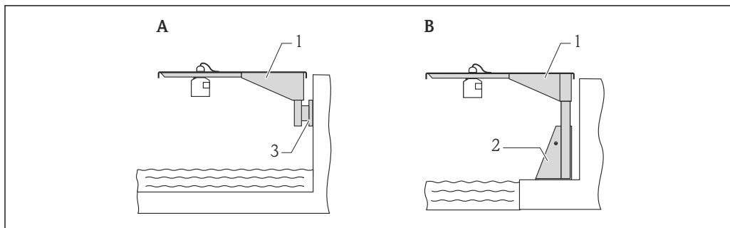
図 14 カンチレバーアームを使用したセンサの取付け
