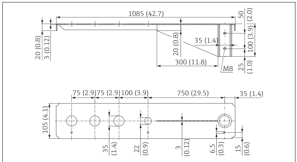
16 寸法。測定単位 mm (in)
