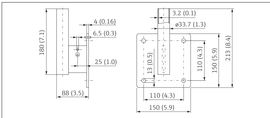
図 19 壁面ブラケットの寸法。測定単位 mm (in)
