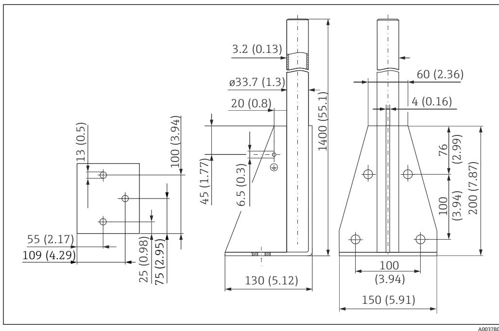
図 18 寸法。測定単位 mm (in)
