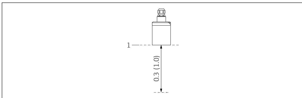
図 1 超音波センサの不感帯：単位 m (ft)
