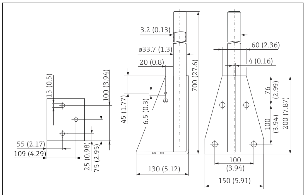
17 寸法。測定単位 mm (in)
