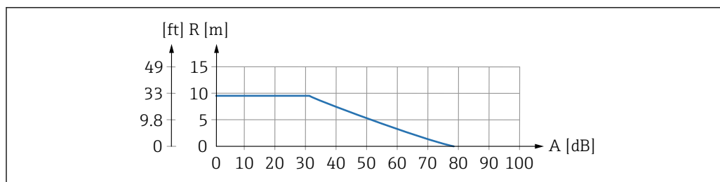
図 2 超音波センサの範囲グラフ
