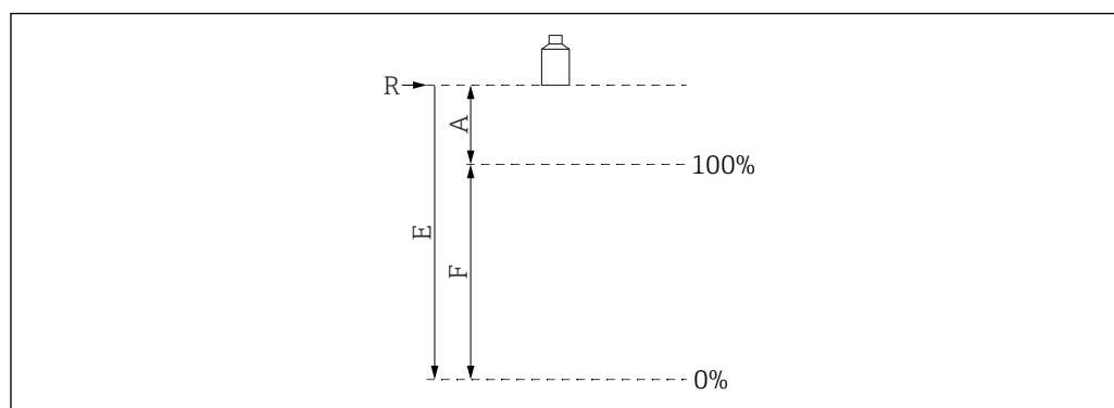
図 12 スパンを定義するための変数
