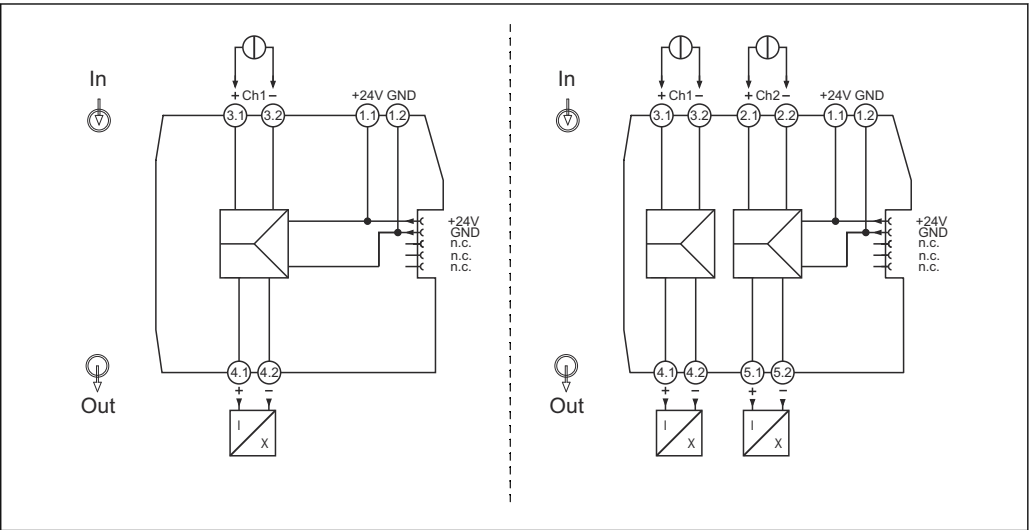
図 8 RNO22 の端子の割当て：1 チャンネルバージョン（左）、2 チャンネルバージョン（右）
