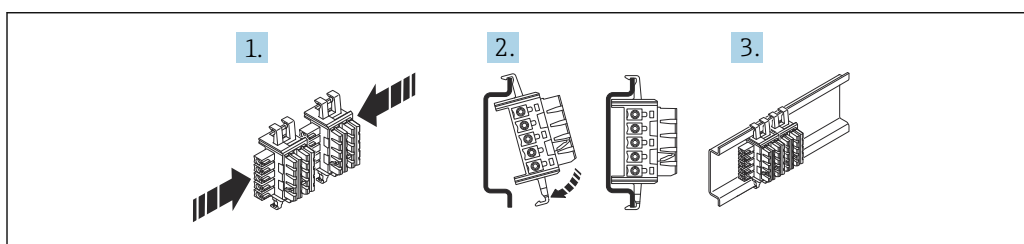
図 2 DIN レールバスコネクタ 12.5 mm (0.5 in) の取付け
