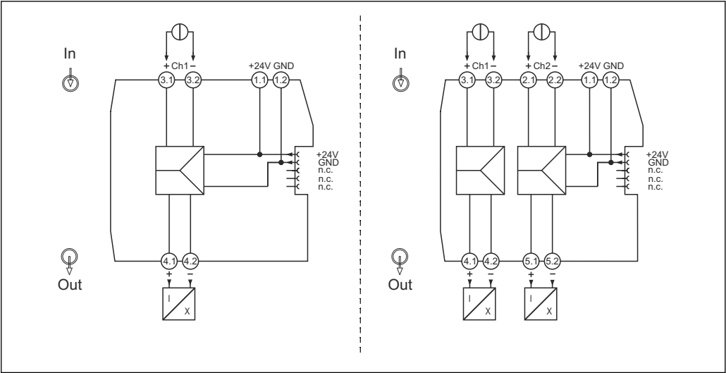
図 6 RNO22 の端子の割当て：1 チャンネルバージョン（左）、2 チャンネルバージョン（右）
