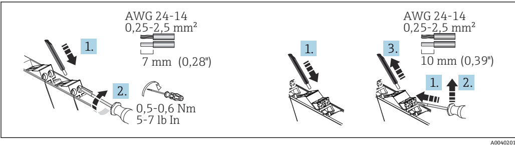
図 9 ネジ端子（左）およびプッシュイン端子（右）を使用した電気接続
