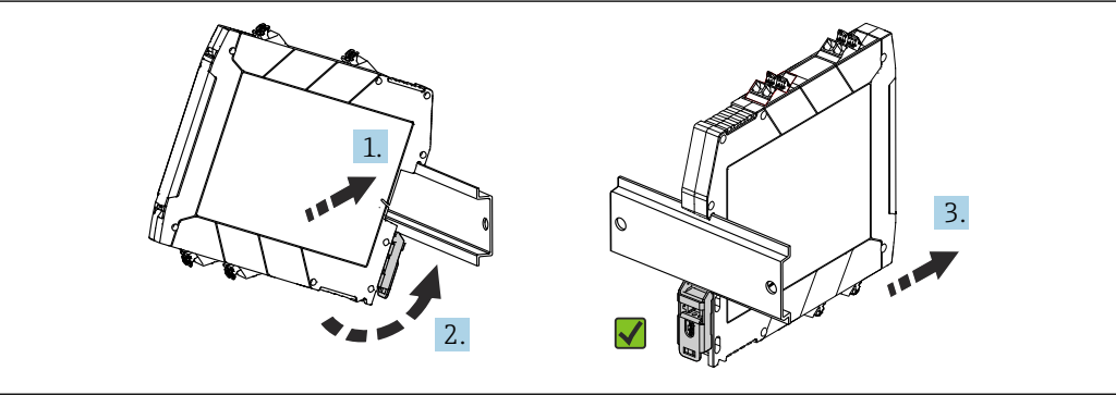
図 10 DIN レールへの取付け
