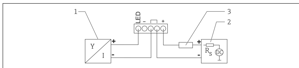
図 6 HART 機器と RIA15 プロセス表示器の接続（ライトあり）
