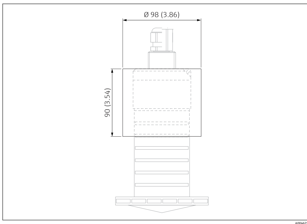
図 35 日除けカバーの寸法、単位：mm (in)
