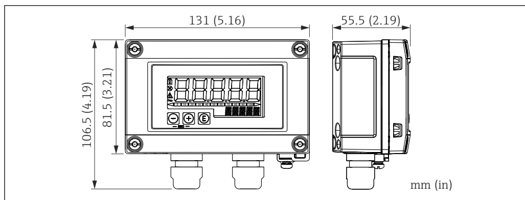
図 51 フィールドハウジング付き RIA15 の寸法、単位：mm (in)
