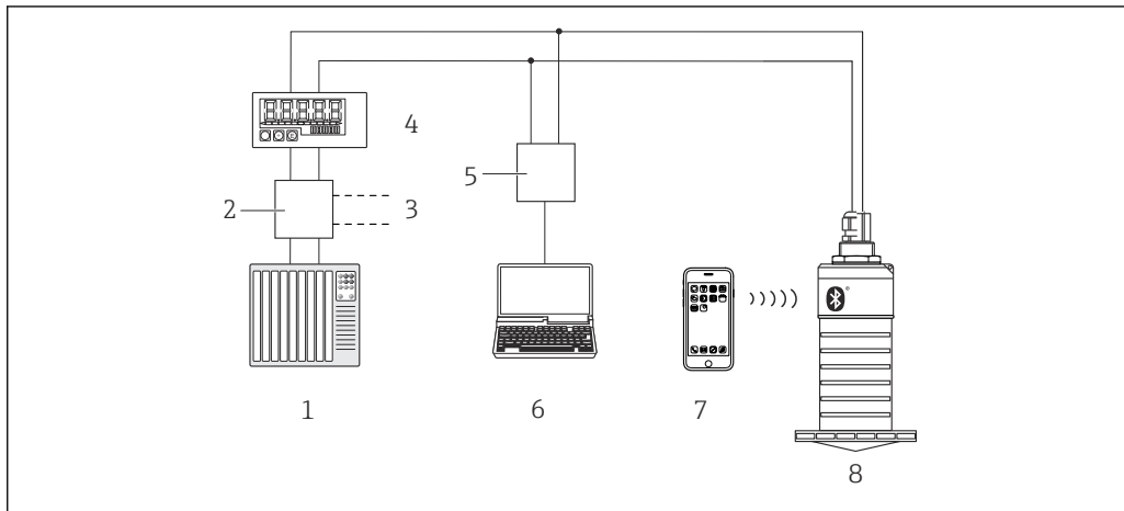
図 34 HART 経由のリモート操作オプション
