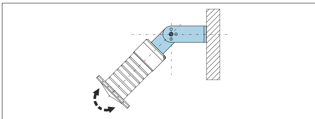
図 19 調整可能な取付ブラケットによる設置
