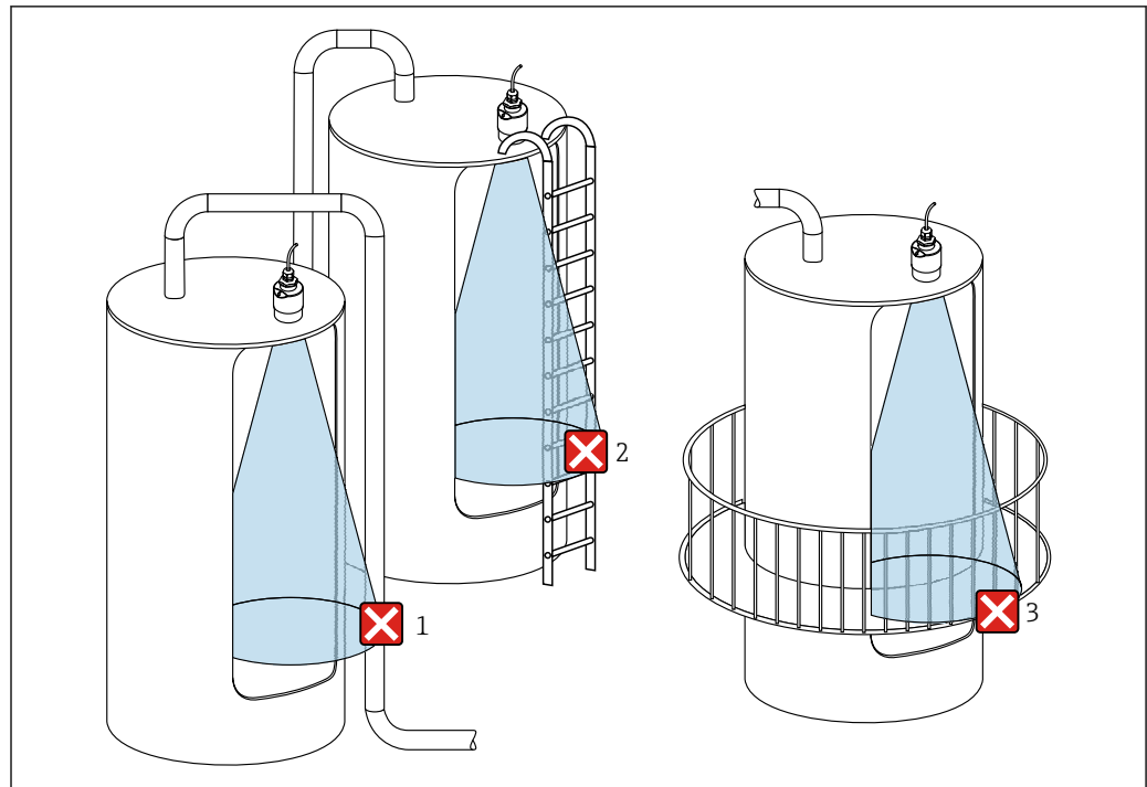
図 16 金属製の干渉物がタンク外側にあるプラスチックタンク内の測定
