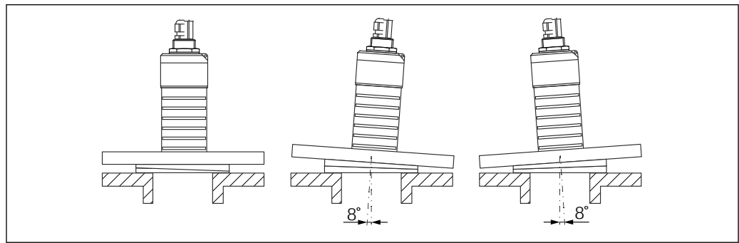
図 24 可変フランジシール付き Micropilot FMR20
