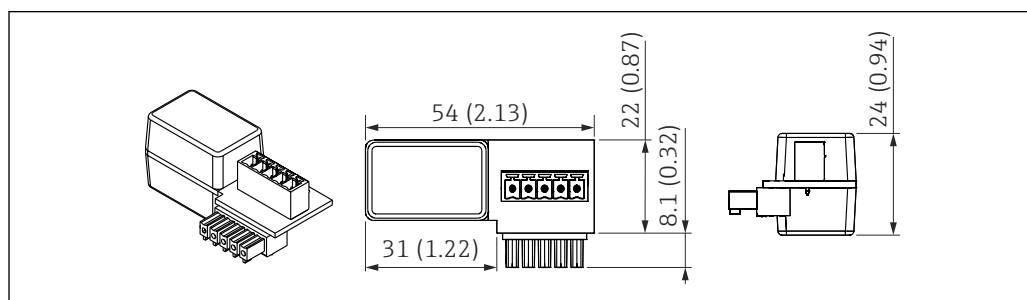
図 52 HART 通信抵抗器の寸法、単位：mm (in)
