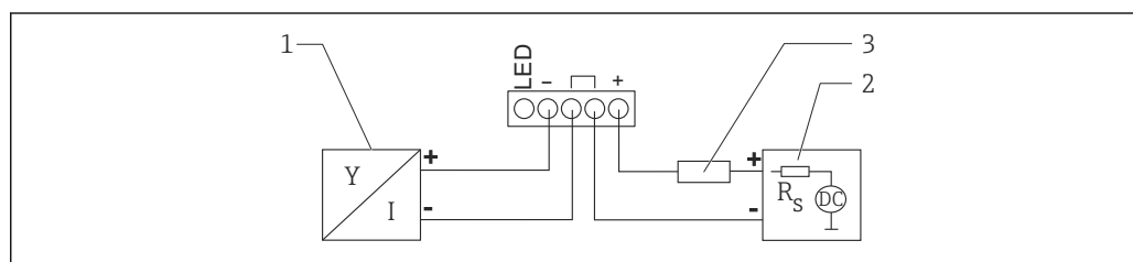
図 5 HART 機器と RIA15 プロセス表示器の接続（ライトなし）
