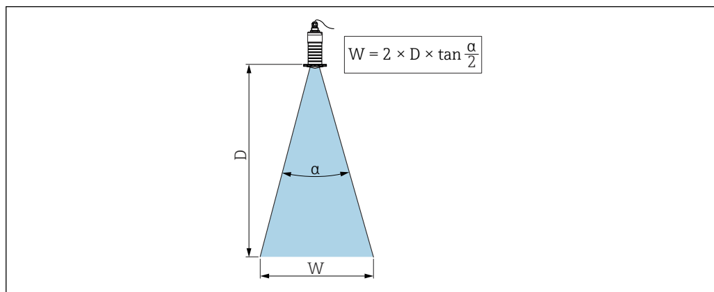
図 15 ビーム放射角 α、距離 D、ビーム幅 W の関係
