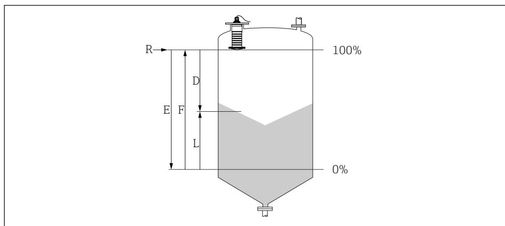
図 1 Micropilot のパラメータの設定
