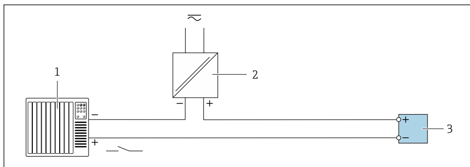
19 Ejemplo de conexión de entrada de estado
