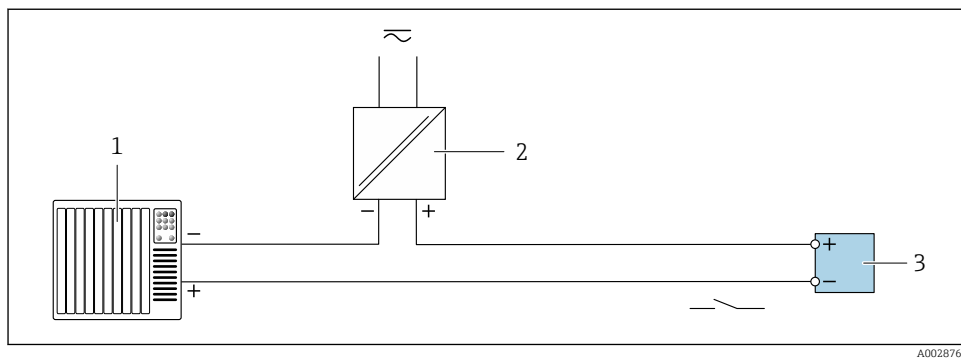
18 Ejemplo de conexión de una salida de conmutación (pasiva)
