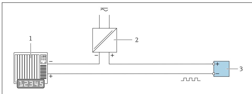
17 Ejemplo de conexión para salida de pulsos/frecuencia (pasiva)
