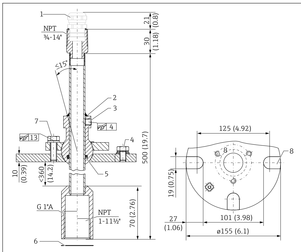
14 Naravni zgib FAU40. Merska enota mm (in)
