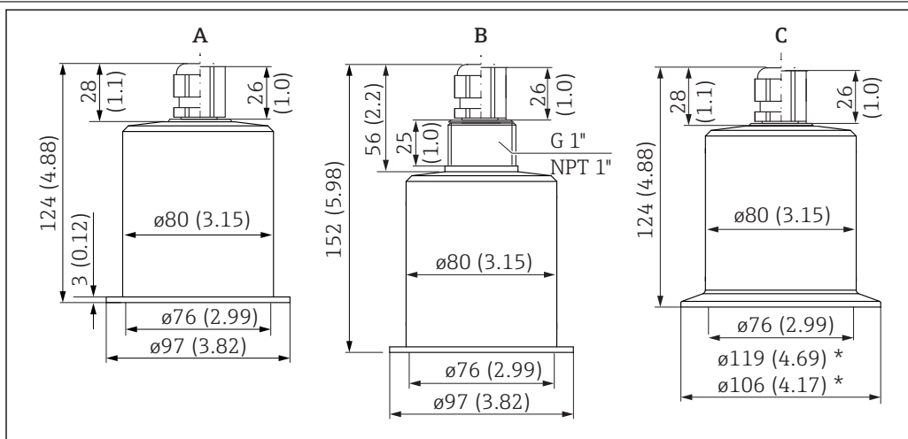
10 Dimenzije. Merska enota mm (in)
