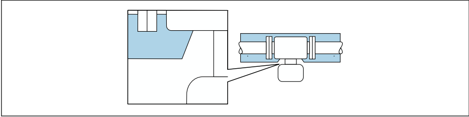
■ 12 단열재가 없는 확장 네크
