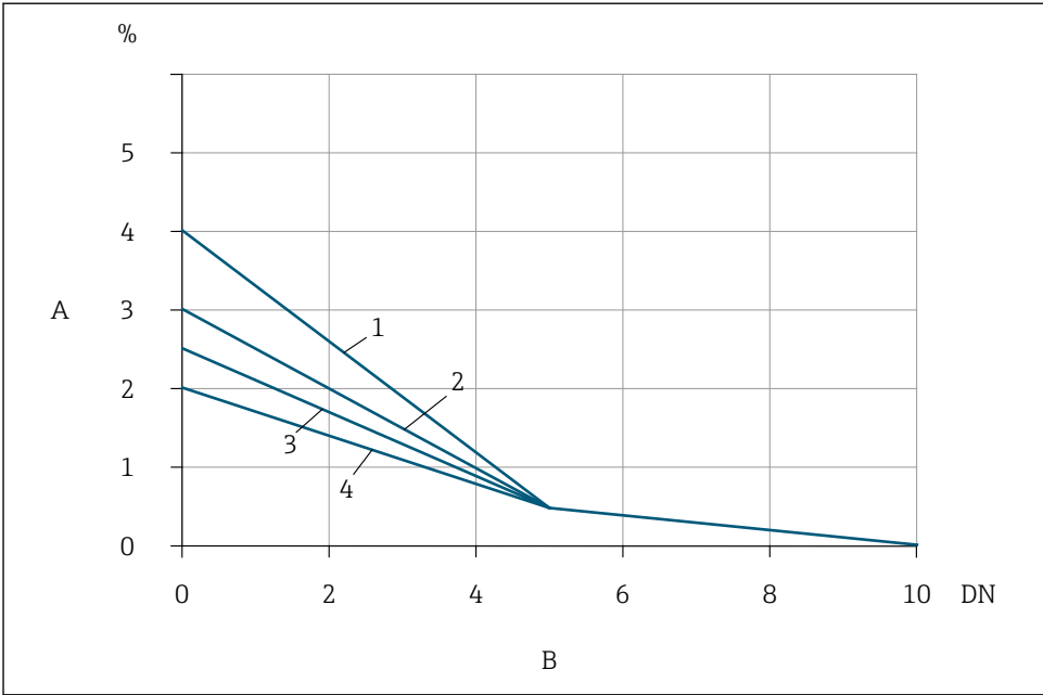
☞ 10 간섭 유형과 전단 직관부에 따라 유량 조절기가 있을 경우 예상되는 추가 측정 오차
