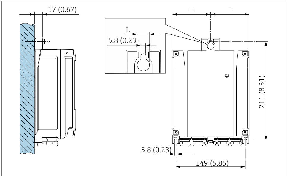
■ 16 공학 단위 mm (in)
