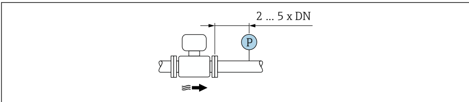
☞ 11 압력 측정 포인트 설치(P = 압력 트랜스미터)
