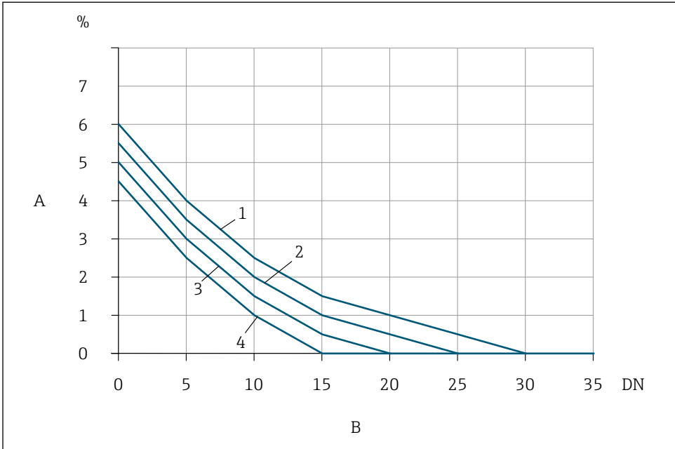
☞ 8 간섭 유형과 전단 직관부에 따라 유량 조절기가 없을 경우 예상되는 추가 측정 오차
