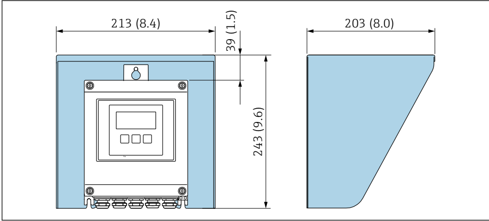
■ 14 Proline 500용 내후성 커버; 공학 단위 mm (in)
