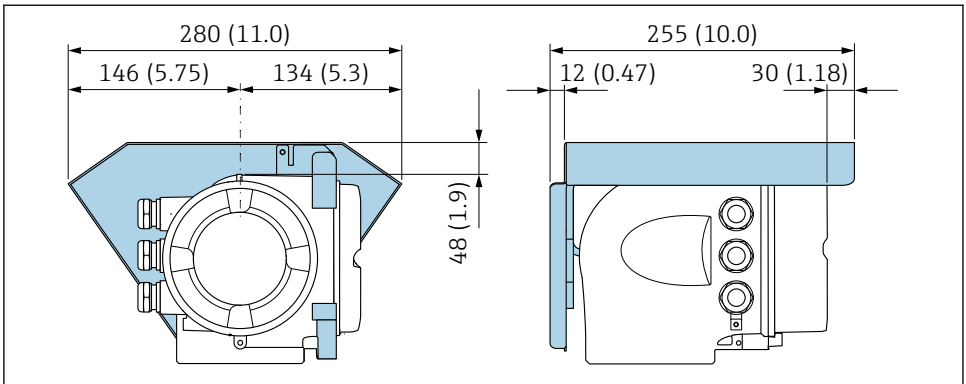
13 공학 단위 mm(in)
