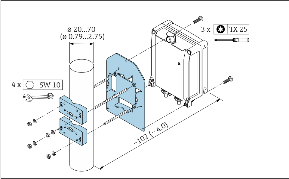
15 공학 단위 mm (in)
