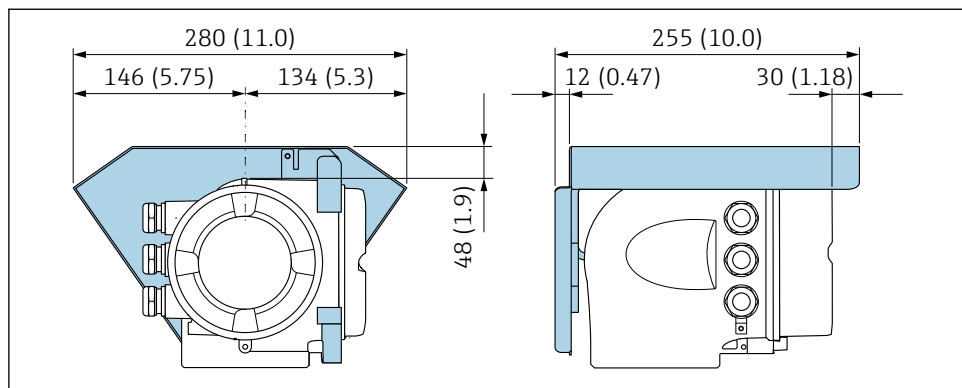
13 Unitate tehnologică mm (in)
