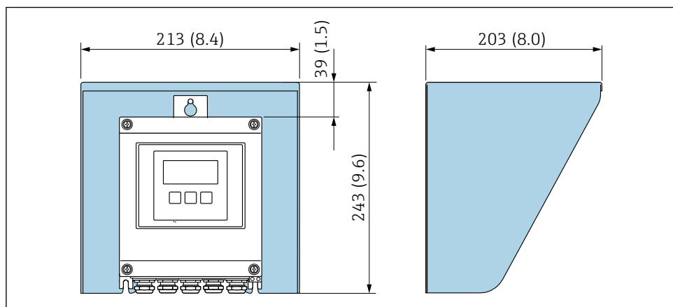
14 Carcasă de protecție împotriva intemperțiilor pentru Proline 500; unitate tehnologică mm (in)
