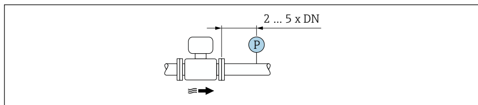
11 Instalarea unui punct de măsurare a presiunii (P = transmițător de presiune)
