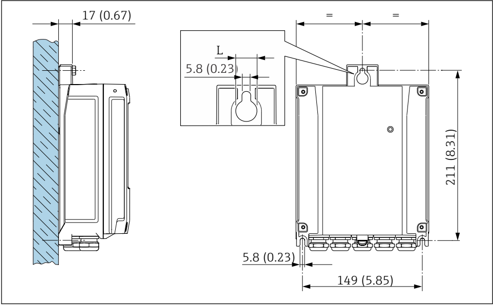
16 Unitate tehnologică mm (in)
