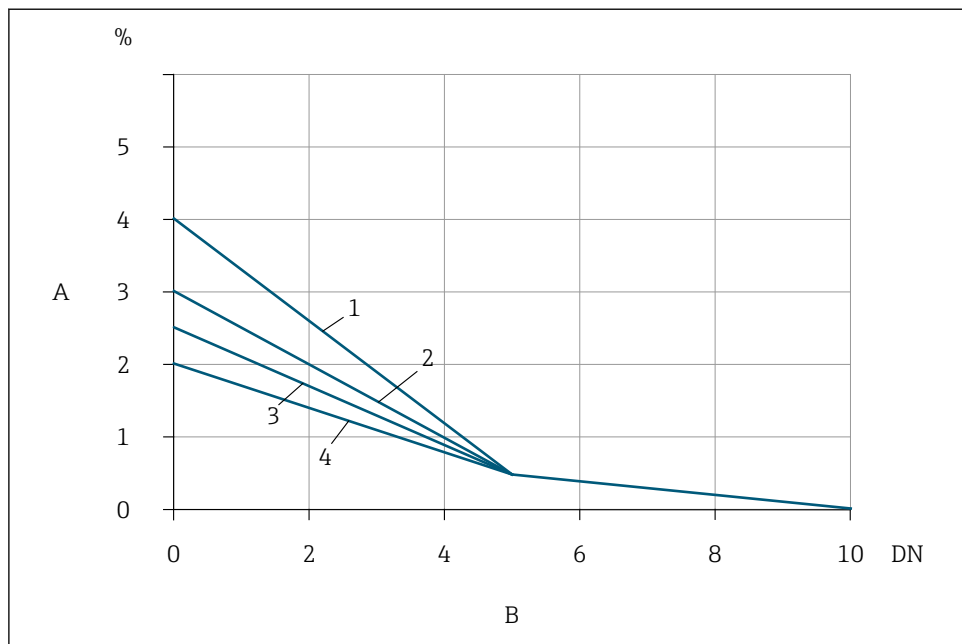
10 Eroarea măsurată suplimentară preconizată cu adaptoare de debit, în funcție de tipul de interferență și de traseul de admisie
