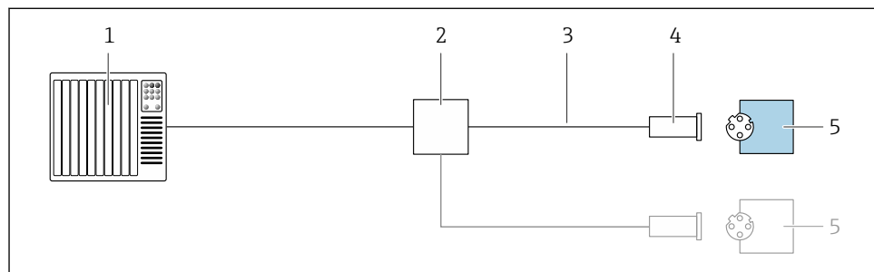
16 Aansluitvoorbeeld voor EtherNet/IP
