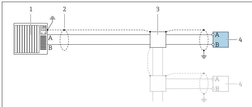
16 Ejemplo de conexión para Modbus RS485, área exenta de peligro y Zona 2/Div. 2
