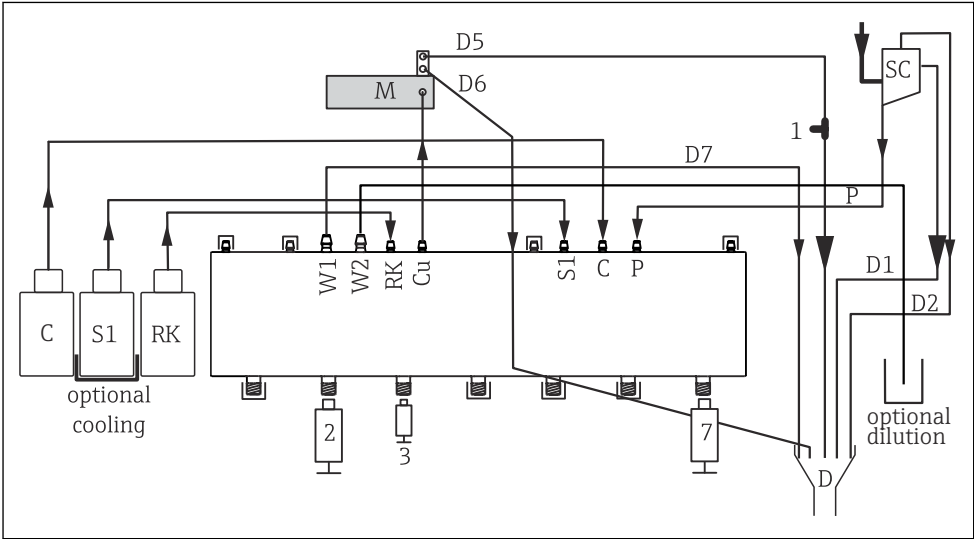
23 Liquiline System CA80NO、1 チャンネル機器
