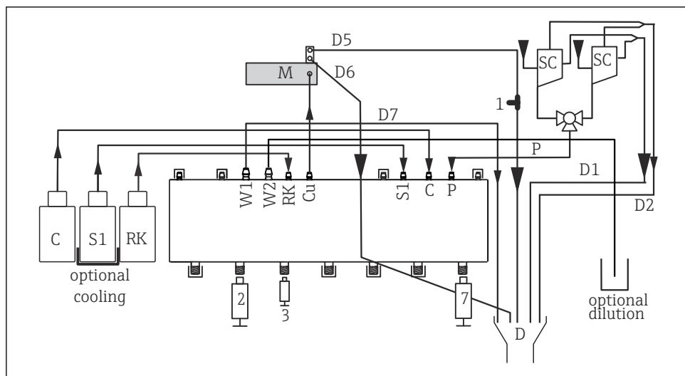
24 Liquiline System CA80NO、2 チャンネル機器
