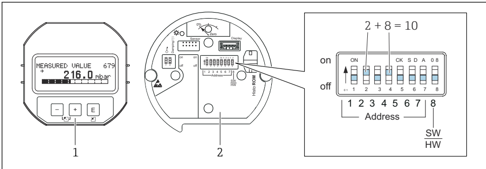
Fig. 8: Ajuste de la dirección del equipo mediante microinterruptores
