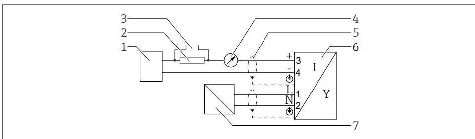
11 Блок-схема, 4-проводное подключение: 4 до 20 мА HART (90 до 253 В АС )
