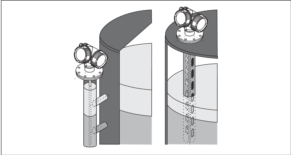
1 Posición de montaje del Levelflex FMP55
