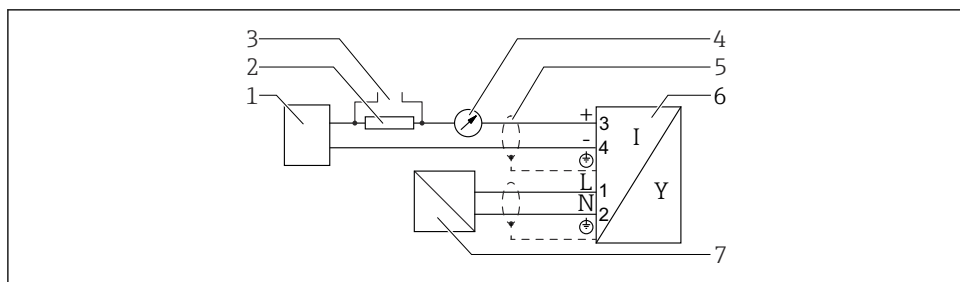
11 Блок-схема, 4-проводное подключение: 4 до 20 мА HART (90 до 253 В AC )
