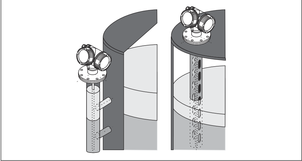
☞ 1 Levelflex FMP55의 설치 위치
