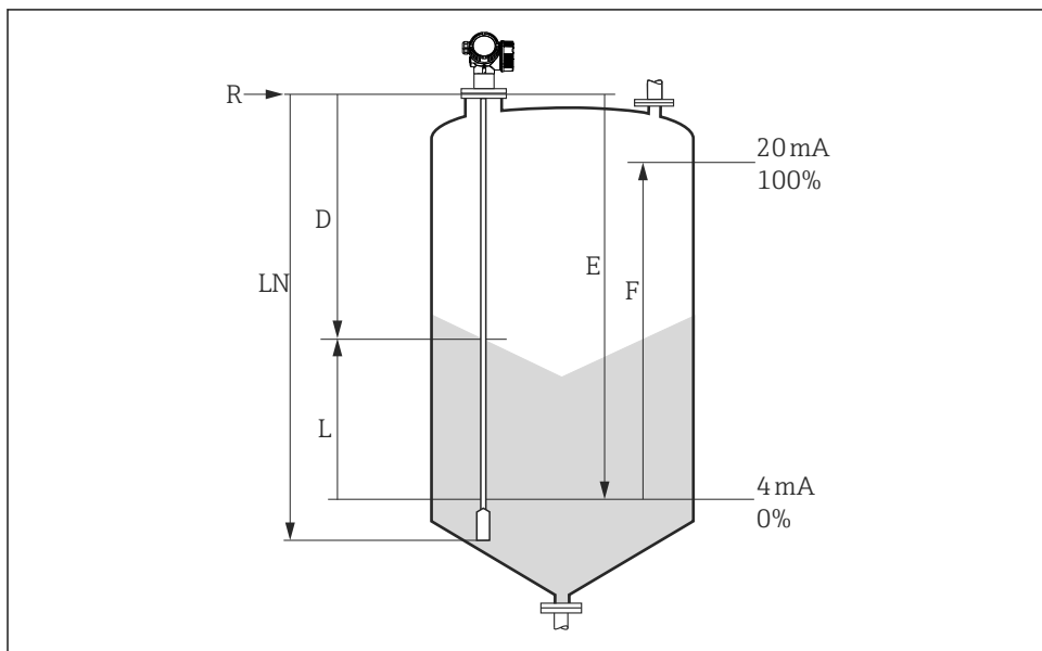
図 11 粉体のレベル測定用パラメータの設定
