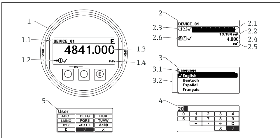
図 8 表示モジュールおよび操作モジュールの表示形式
