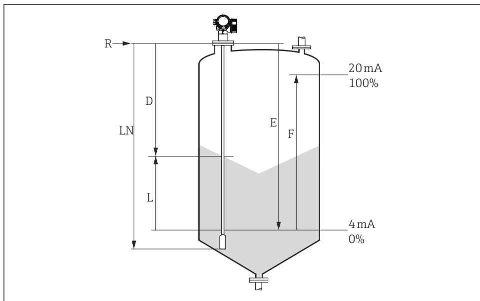
11 Parametry konfiguracyjne pomiaru poziomu materiałów sypkich
