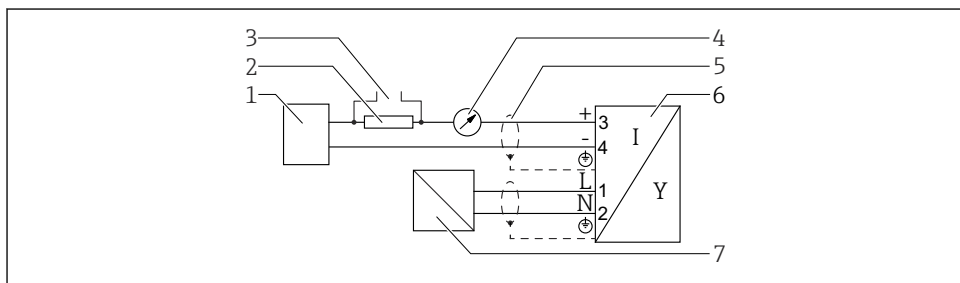
11 Blokdiagram, 4 ledere: 4 til 20 mA HART (90 til 253 V AC )
