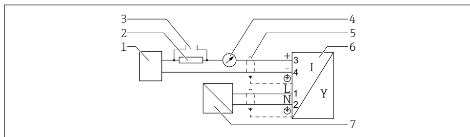
11 Schemat blokowy wersji 4-przewodowej 4 ... 20 mA HART (90 ... 253 V AC )
