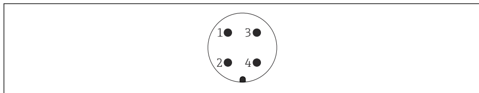
13 Přřazení kontaktů konektoru 7/8"
