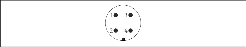
4 Přirazení kontaktů konektoru 7/8"
