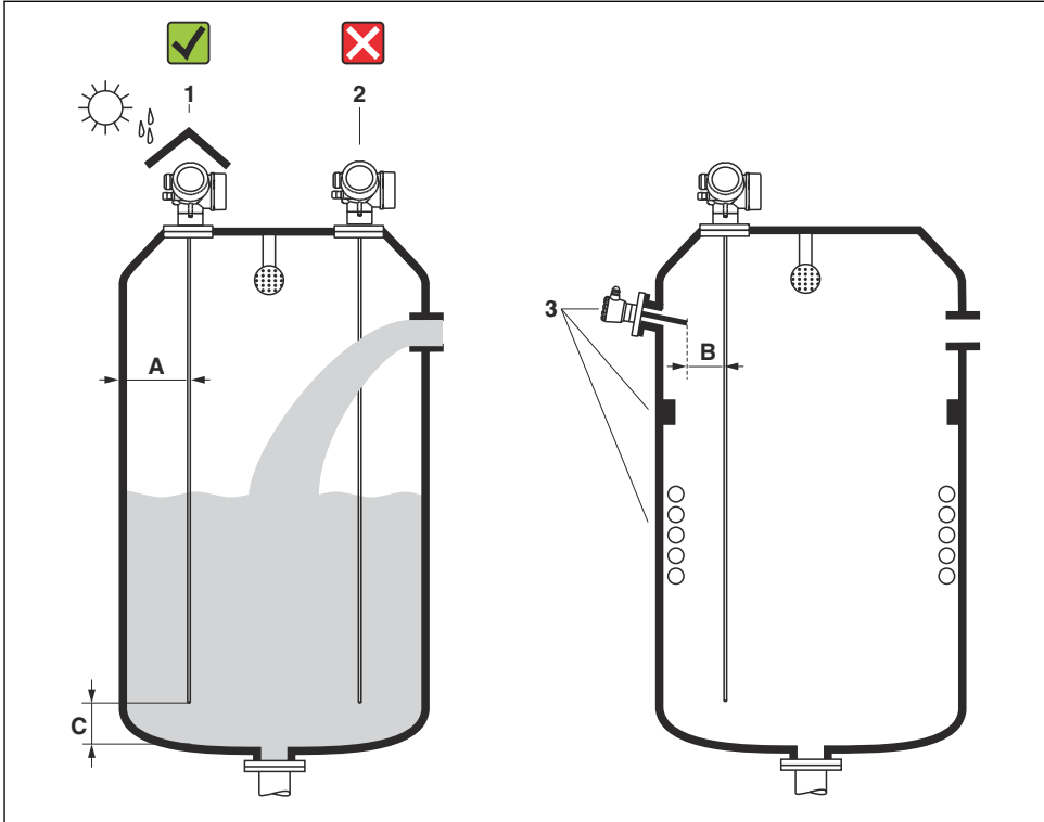
1 Levelflex 설치 조건
