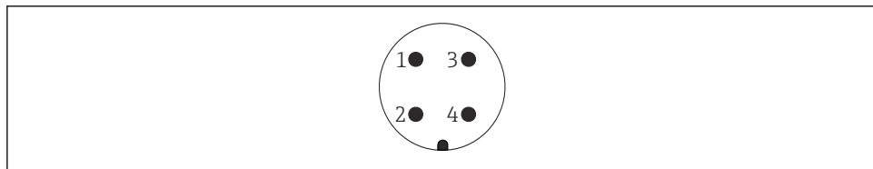
4 Tildeling af ben for 7/8"-stik
