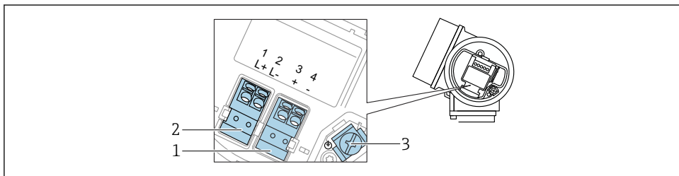
図 9 端子の割当て、4 線式：4～20 mA HART（10.4～48 V DC ）
