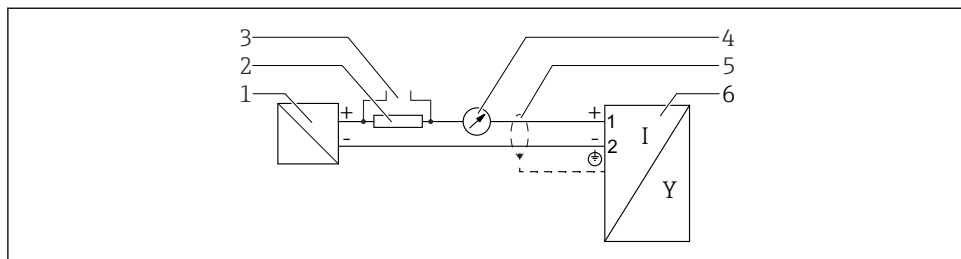
■ 4 ブロック図、2線式：4～20 mA HART
