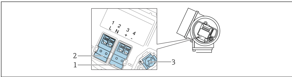
図 11 端子の割当て、4 線式：4～20 mA HART（90～253 V AC ）
