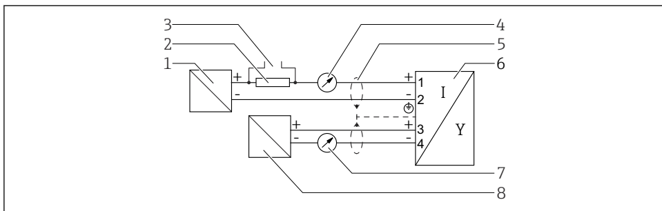
図 8 ブロック図、2 線式：4～20 mA HART、4～20 mA
