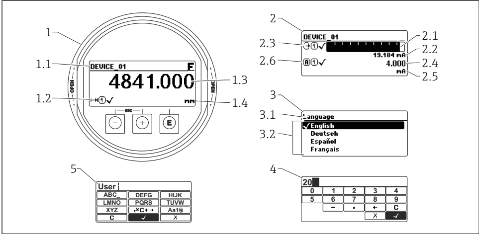
図 18 表示モジュールおよび操作モジュールの表示形式
