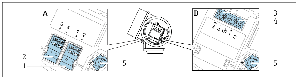
■ 5 端子の割当て、2 線式：4～20 mA HART、スイッチ出力
