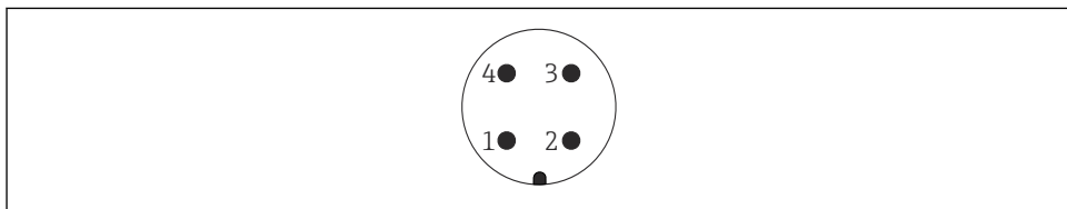
14 Tildeling af ben for M12-stik
