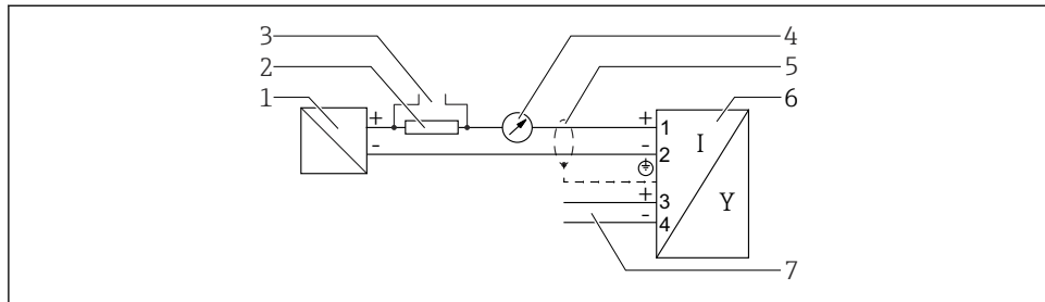
7 Blokkdiagram, 2-leder: 4 – 20 mA HART, bryterutgang
