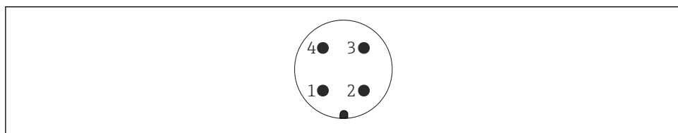
14 Pinnetilordning av M12-plugg
