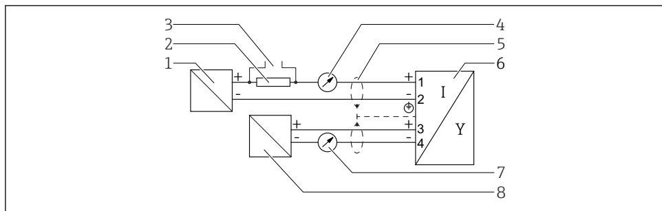
13 Blokkdiagram, 2-vezetékes: 4 ... 20 mA HART, 4 ... 20 mA
