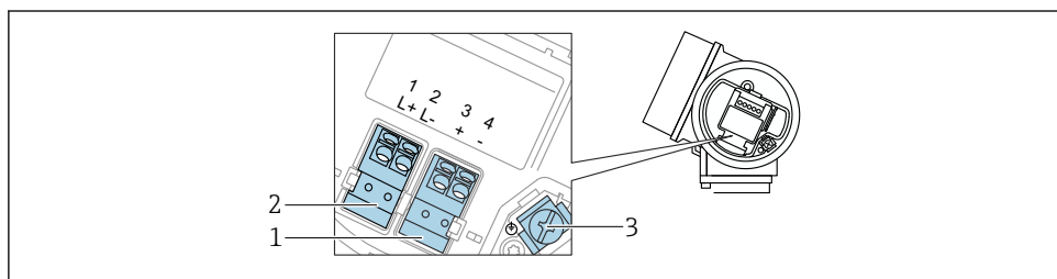
14 Kapocskiosztás, 4-vezetékes: 4 ... 20 mA HART (10.4 ... 48 V DC )
