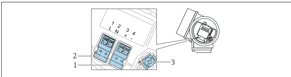
16 Přiřazení svorek, čtyřvodič: 4 ... 20 mA HART (90 ... 253 V AC )
