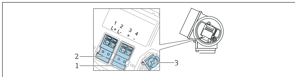
14 Přiřazení svorek, čtyřvodič: 4 ... 20 mA HART (10,4 ... 48 V DC )
