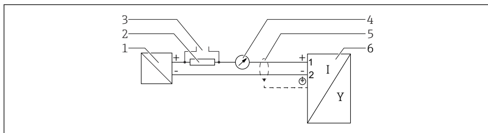
9 Blokové schéma, dvojvodič: 4 ... 20 mA HART
