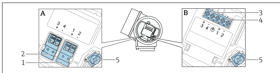
10 Přiřazení svorek, dvojvodič: 4 ... 20 mA HART, spínaný výstup
