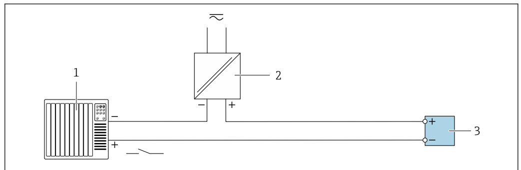
21 ステータス入力の接続例
