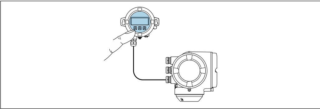
43 分離型ディスプレイと操作モジュール DKX001 を介した操作
