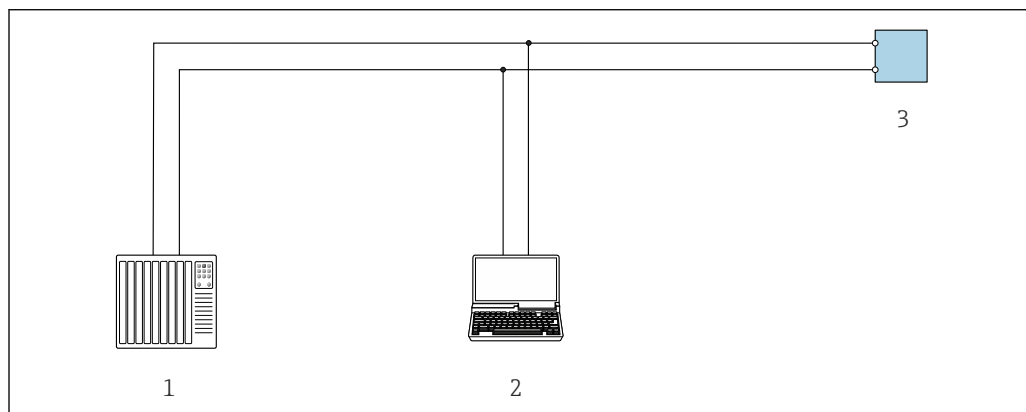
図 49 Modbus-RS485 プロトコル経由のリモート操作オプション（アクティブ）
