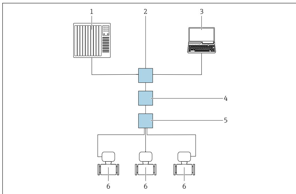
図 54 APL ネットワーク経由のリモート操作用オプション
