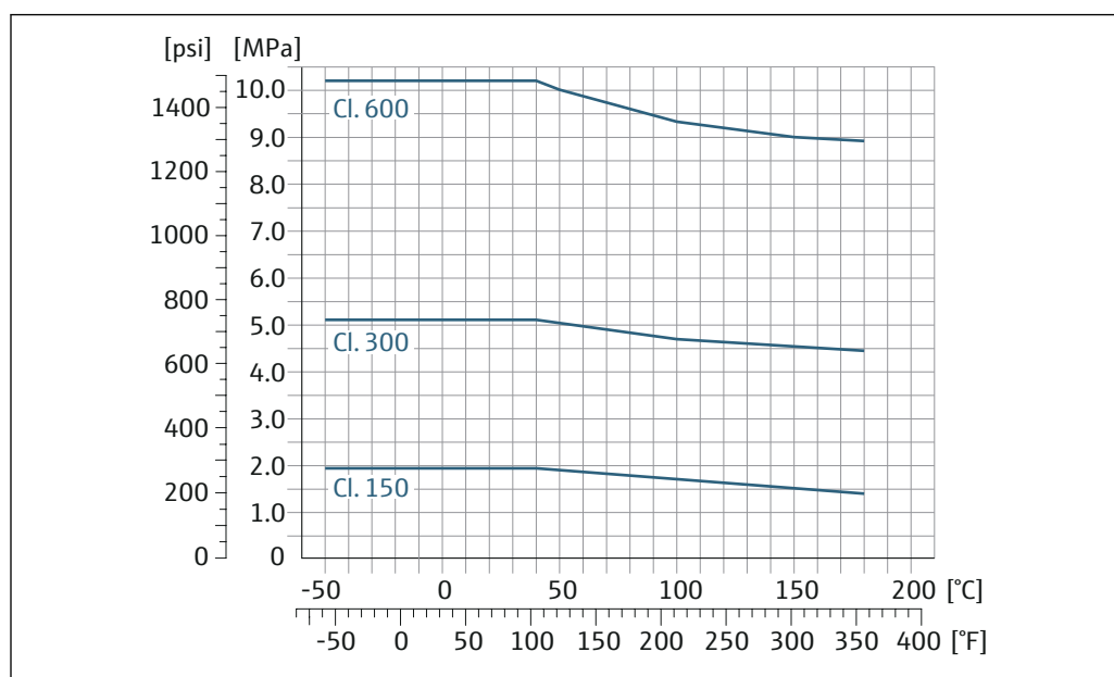
図 27 フランジ材質 1.4404 (SUS 316 または 316L 相当)
