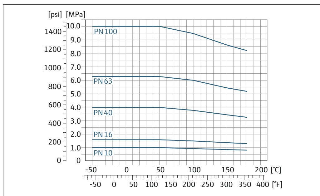
図 26 フランジ材質 1.4404 (SUS 316 または 316L 相当)
