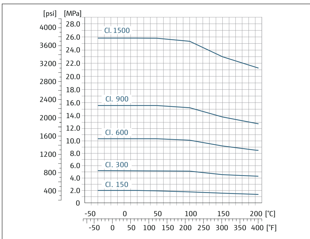
図 32 フランジ材質：ステンレス 1.4410/F53 25Cr 二相（スーパー二相）
