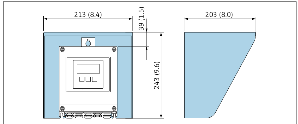
36 Proline 500 – デジタル用の日除けカバー、単位 mm (in)
