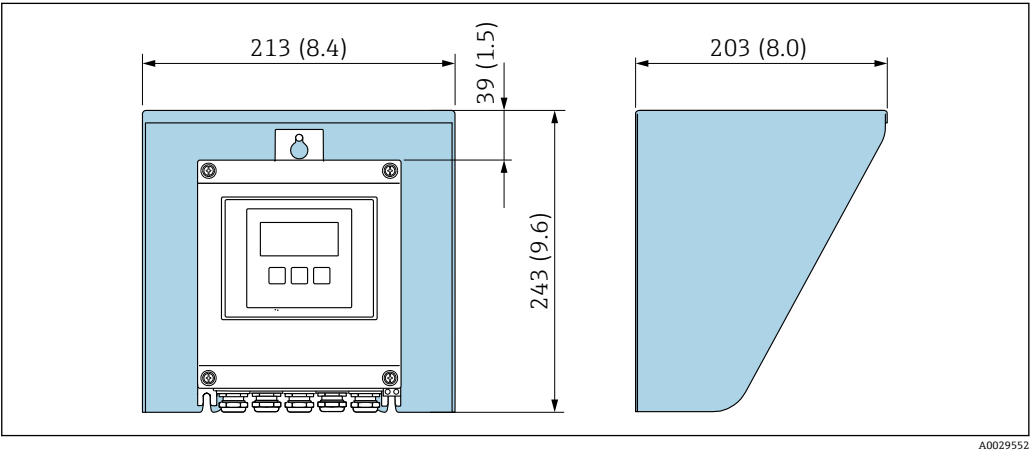
42 Proline 500 – デジタル用の日除けカバー、単位 mm (in)
