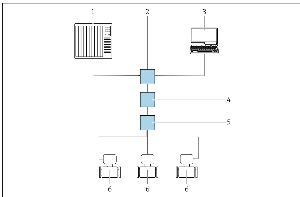
図 60 APL ネットワーク経由のリモート操作オプション
