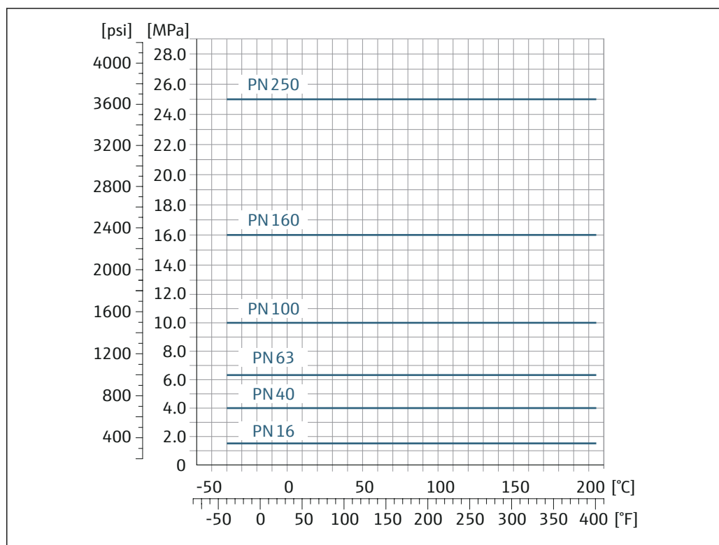
図 31 フランジ材質：ステンレス 1.4410/F53 25Cr 二相（スーパー二相）
