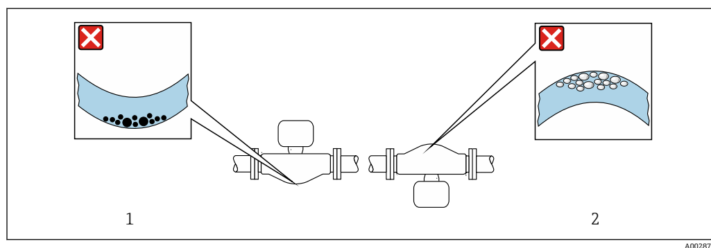
☒ 23 弓形計測チューブセンサの取付方向
