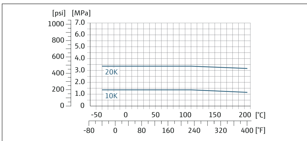
図 33 フランジ材質：ステンレス 1.4410/F53 25Cr 二相（スーパー二相）
