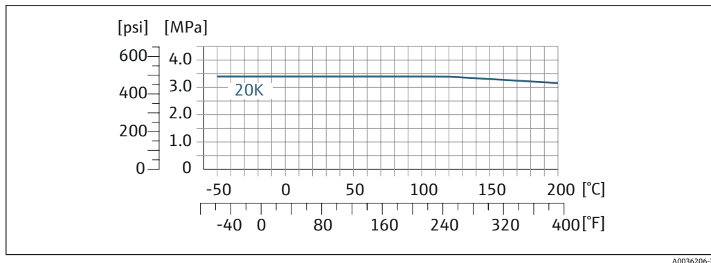
37 ラップジョイントフランジ、フランジ材質：1.4301 (SUS F304 相当)、接液部 アロイ C22 : 2.4602 (UNS N06022)
