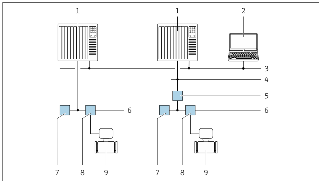
図 58 FOUNDATION フィールドバスネットワークを介したリモート操作のオプション
