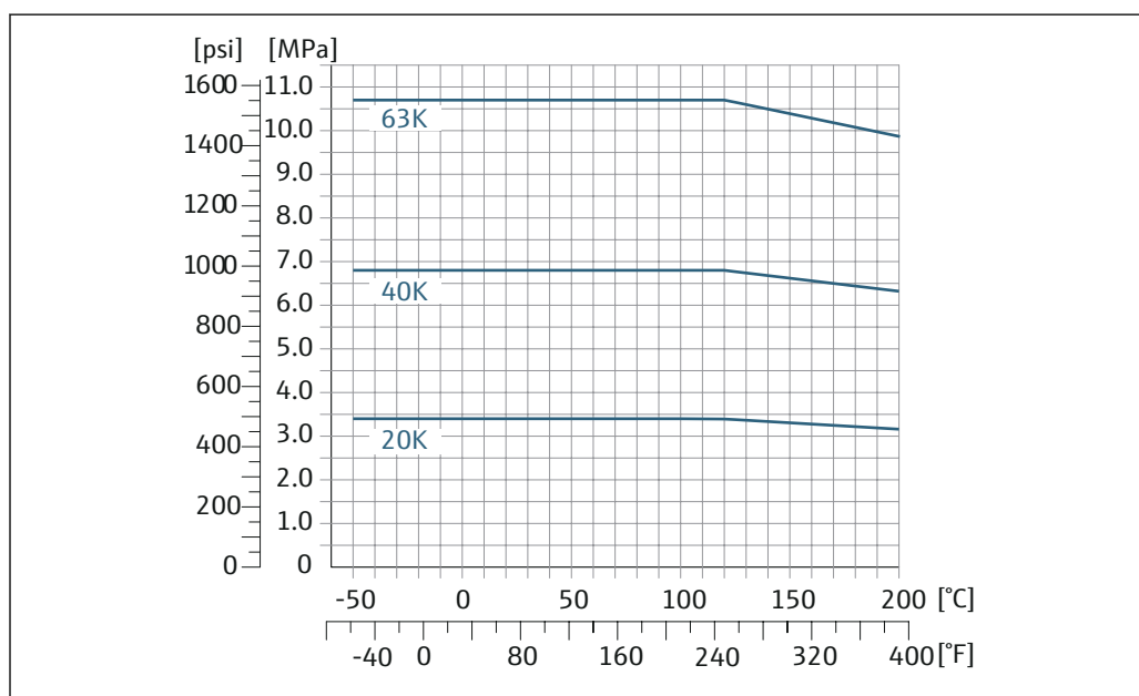
図 36 フランジ材質：1.4404 (SUS 316 または 316L 相当) またはアロイ C22、2.4602 (UNS N06022)
