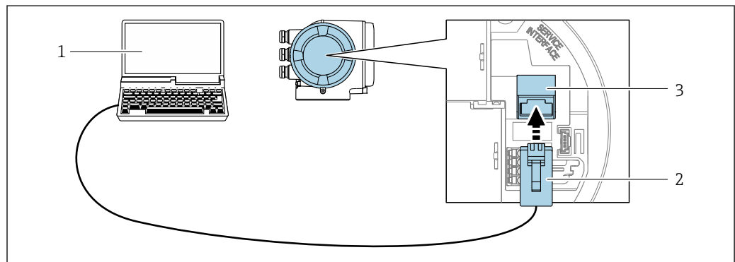
図 68 サービスインターフェイス (CDI-RJ45) 経由の接続
