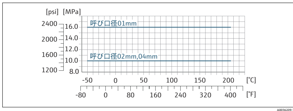
38 フランジ材質：1.4404 (SUS 316 または 316L 相当)
