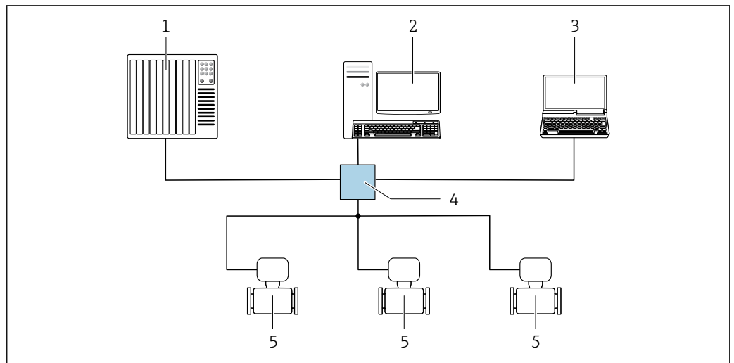
図 62 EtherNet/IP ネットワーク経由のリモート操作用オプション：スター型トポロジー
