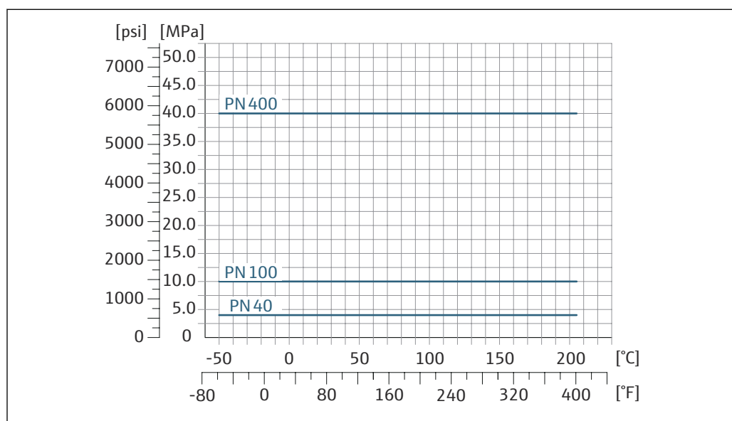
図 31 フランジ材質：アロイ C22、2.4602 (UNS N06022)
