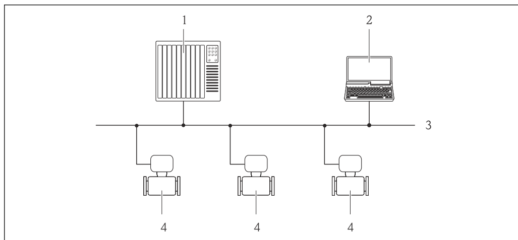
図 59 PROFIBUS DP ネットワークを介したリモート操作のオプション
