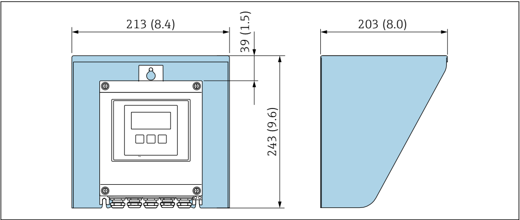
42 Proline 500 – デジタル用の日除けカバー、単位 mm (in)
