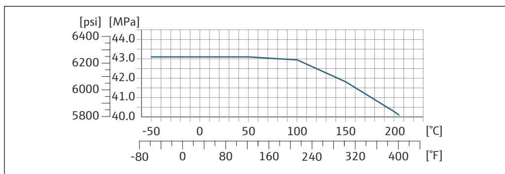
図 40 フランジ材質：アロイ C22、2.4602 (UNS N06022)；「計測チューブの材質、接液部表面」のオーダーコード、オプション HB
