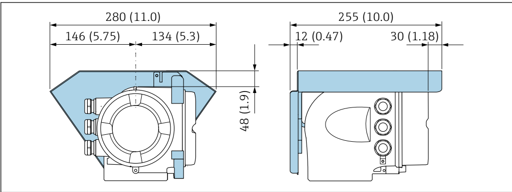
図 28 Proline 500 用の日除けカバー、単位 mm (in)
