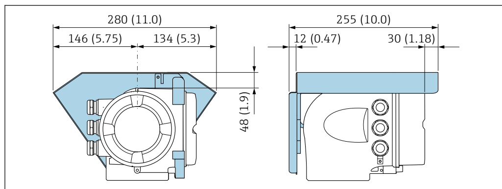
図 49 Proline 500 用の日除けカバー、単位 mm (in)
