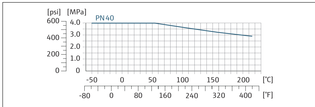
32 ラップジョイントフランジ、フランジ材質：1.4301 (SUS F304 相当)、接液部 アロイ C22 : 2.4602 (UNS N06022)
