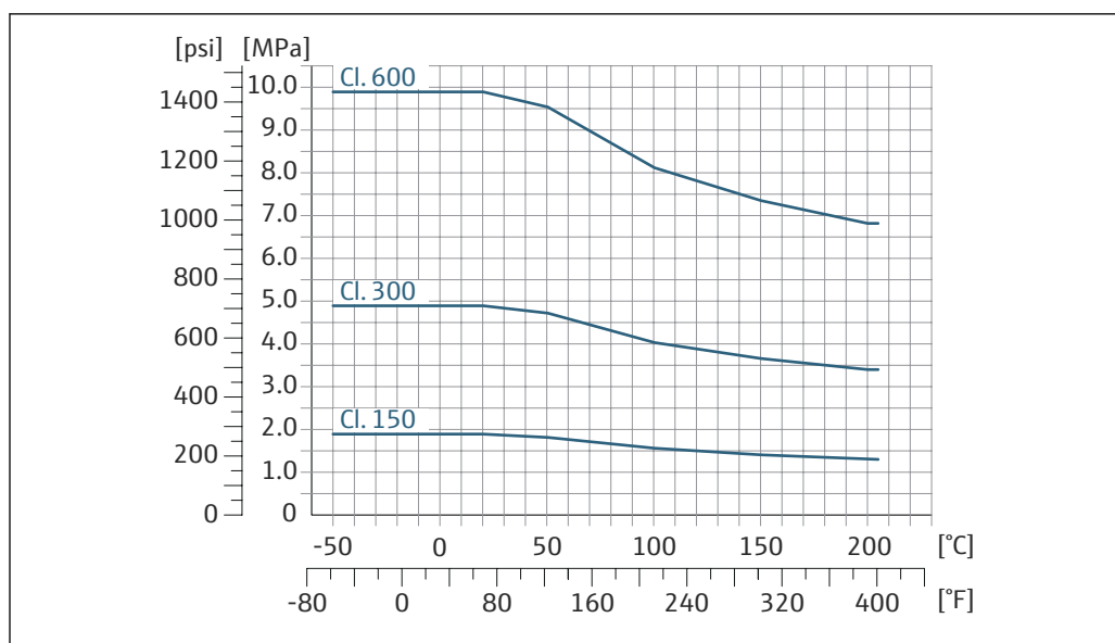
図 35 ラップジョイントフランジ、フランジ材質：1.4301 (SUS F304 相当)、接液部 アロイ C22 : 2.4602 (UNS N06022)
