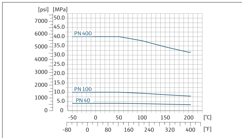
図 30 フランジ材質：1.4404 (SUS 316 または 316L 相当)
