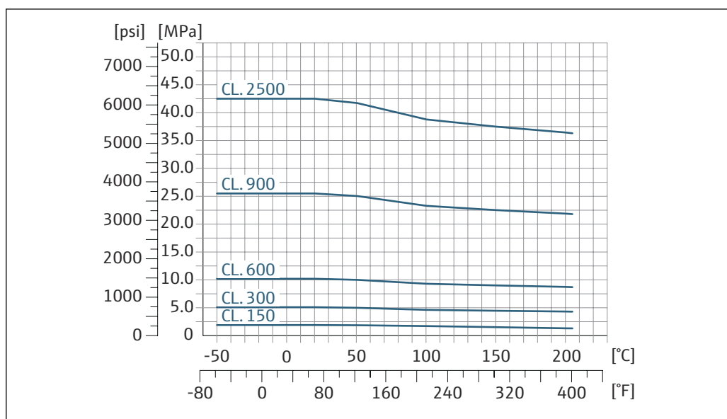
33 フランジ材質：1.4404 (SUS 316 または 316L 相当)
