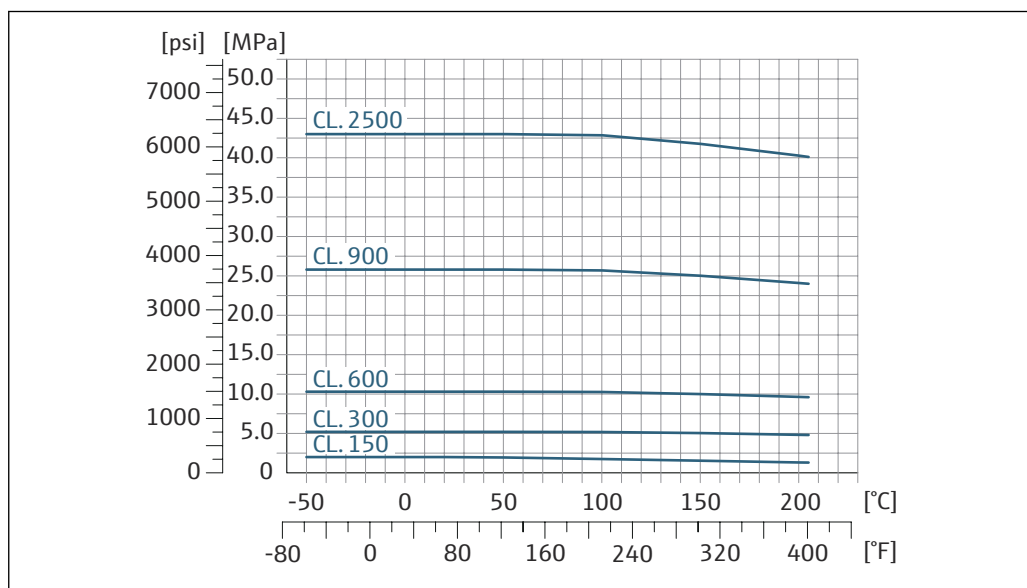
34 フランジ材質：アロイ C22、2.4602 (UNS N06022)
