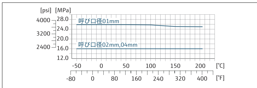
39 フランジ材質：アロイ C22、2.4602 (UNS N06022)
