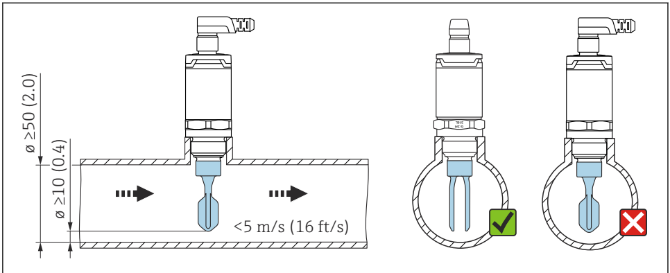
図 8 パイプ内の音叉部の位置。測定単位 mm (in)
