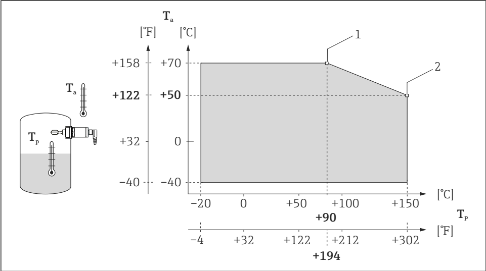
18 ディレーティング曲線：150 ^{\circ}\text{C} (302 ^{\circ}\text{F} )
