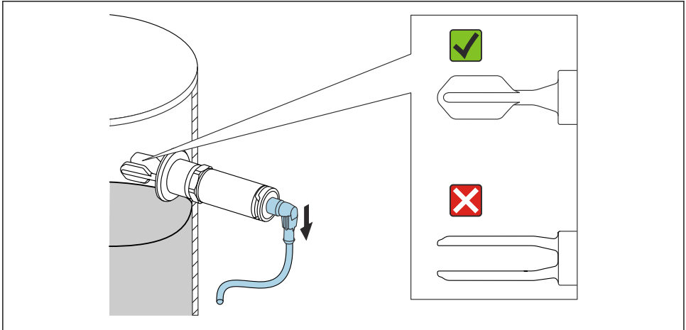
図 9 水平設置時の容器内の音叉フォークの位置
