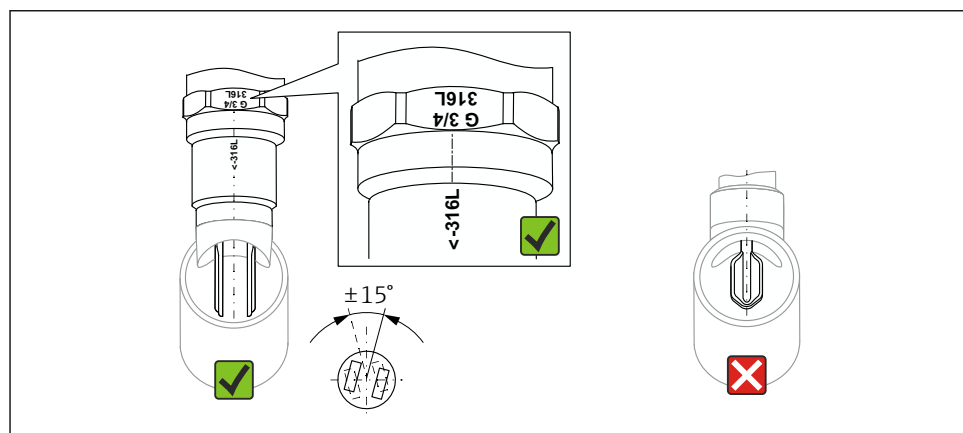
図 7 パイプ内での方向
