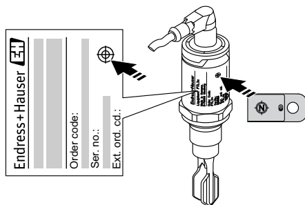
図 16 ハウジングに対するテストマグネットの位置
