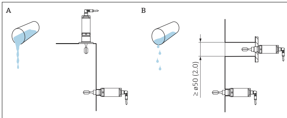
図 4 液体粘度を考慮した設置オプション (寸法単位 : mm (in))
