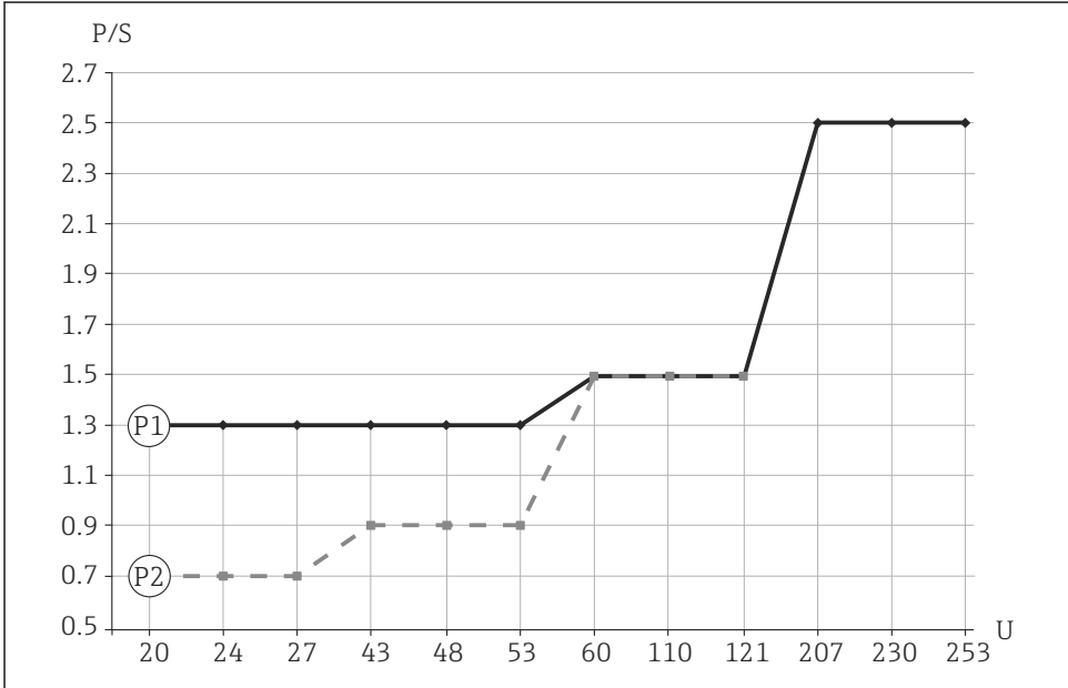
図 13 負荷の最小定格電力
