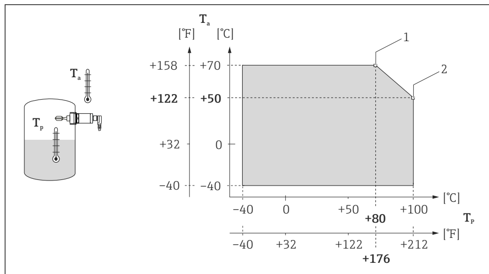
図 17 ディレーティング曲線 : 100 °C (212 °F)
