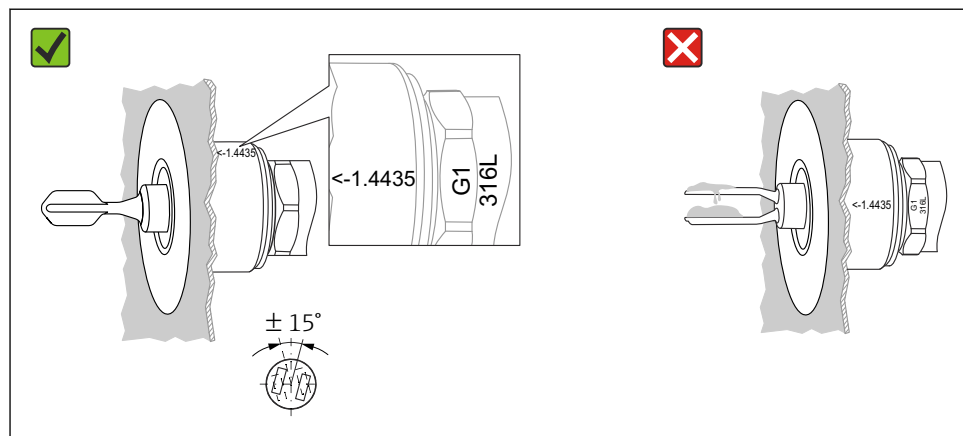
図 6 容器内での方向
