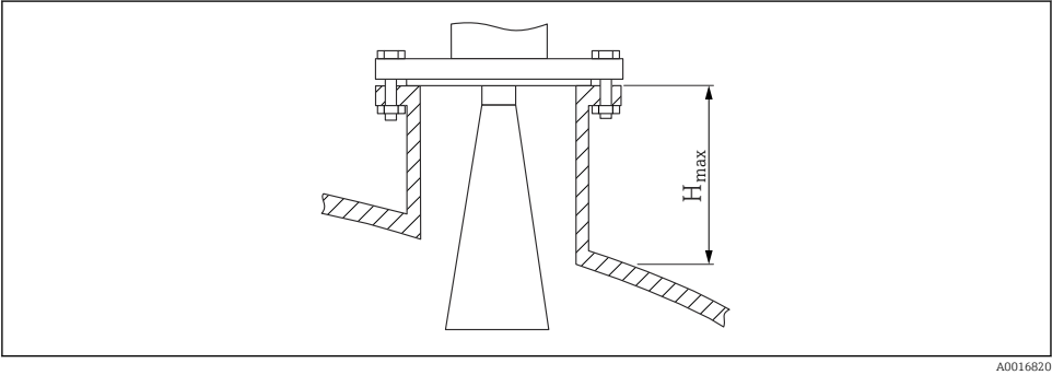
2 Wysokość króćca montażowego dla anteny stożkowej (FMR51)
