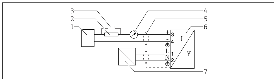
13 Schemat blokowy wersji 4-przewodowej 4 ... 20 mA HART (90 ... 253 V AC )
