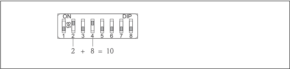
10 Példa hardveres címzésre: a 8-as kapcsoló „OFF” állásban van; az 1–7. kapcsolók határozzák meg a címet.
