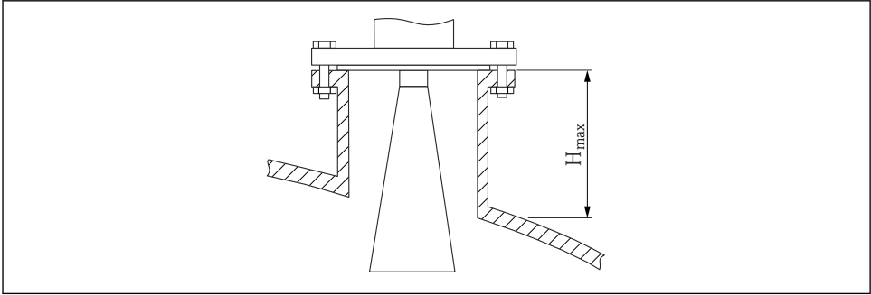
2 Dysehøjde for hornantenne (FMR51)
