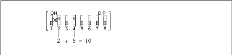
14 Przykład adresacji sprzętowej: mikroprzelącznik 8 w pozycji "OFF"; mikroprzelączniki 1 do 7 służą do ustawienia adresu.
