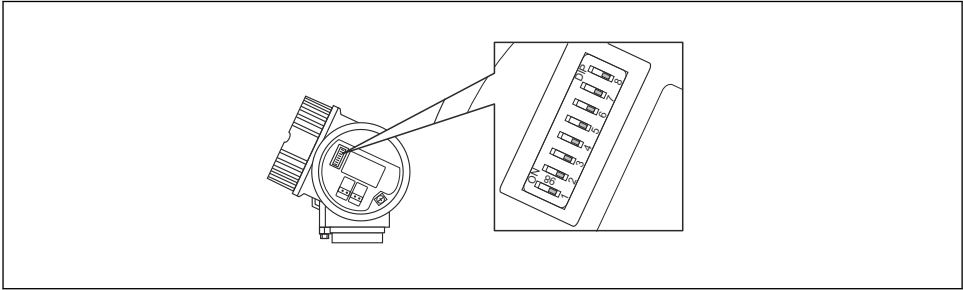
13 Mikroprzelączniki ustawiania adresu w przedziale podłączeniowym
