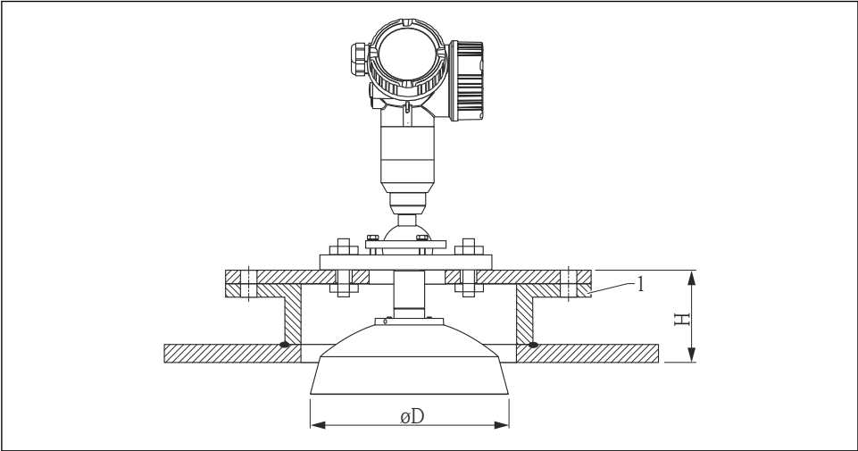
1 Króciec
