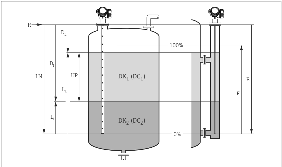
图 19 界面测量设置参数
