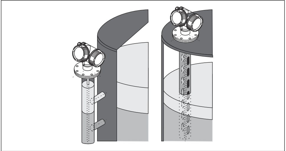
图 1 Levelflex FMP55 的安装位置
