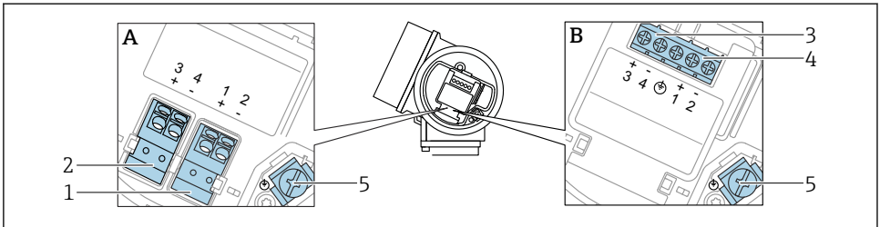
图 6 接线端子分配，两线制：4 ... 20 mA HART，4 ... 20 mA
