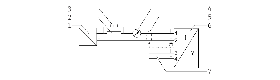
图 5 接线图：两线制：4 ... 20 mA HART，开关量输出
