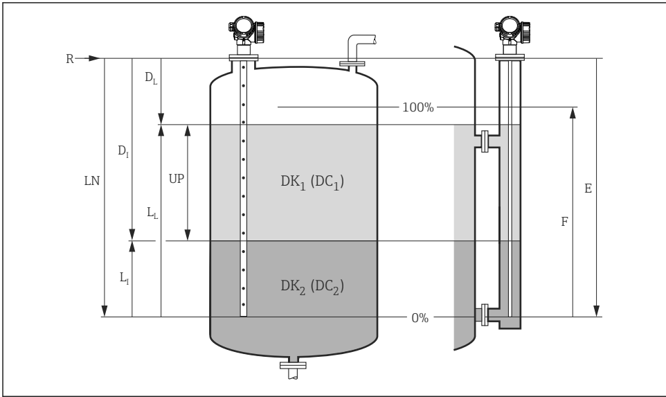
图 10 界面测量设置参数
