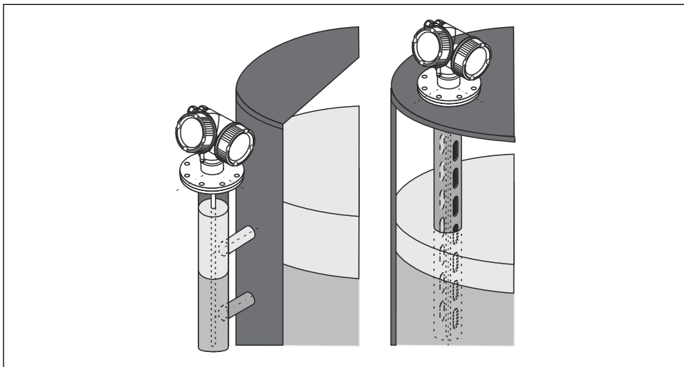
图 1 Levellflex FMP55 的安装位置
