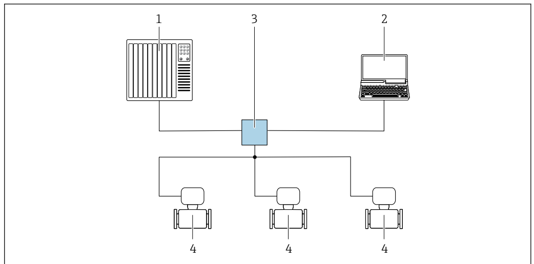
图 54 通过 PROFINET 网络进行远程操作：星形拓扑结构
