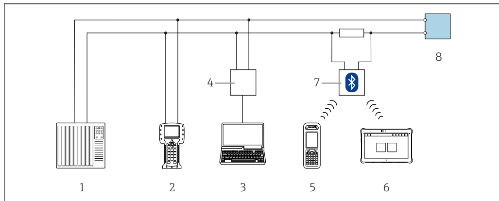
46 通过 HART 通信进行远程操作（有源信号）
