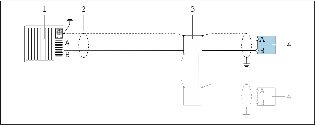
12 接线实例：Modbus RS485，非危险区和防爆 2 区；Cl. I, Div. 2 防爆场合
