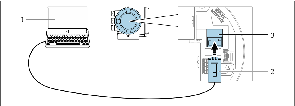
图 57 通过服务接口（CDI-RJ45）连接
