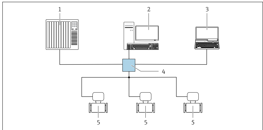
图 52 通过 EtherNet/IP 网络进行远程操作：星形拓扑结构
