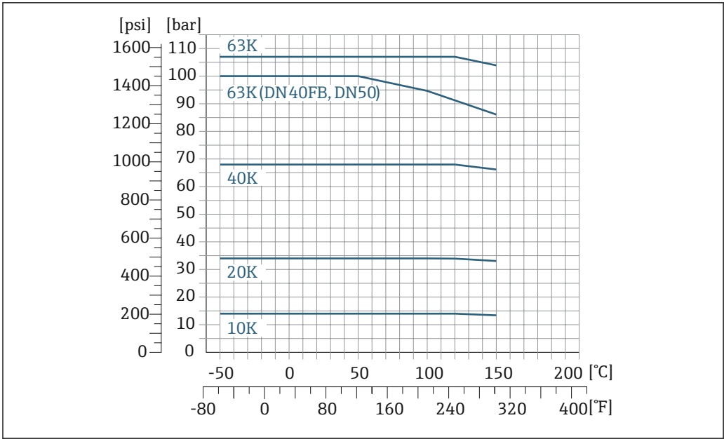
图 27 法兰材质: 1.4301 (304) ; 接液部件材质: 钛
