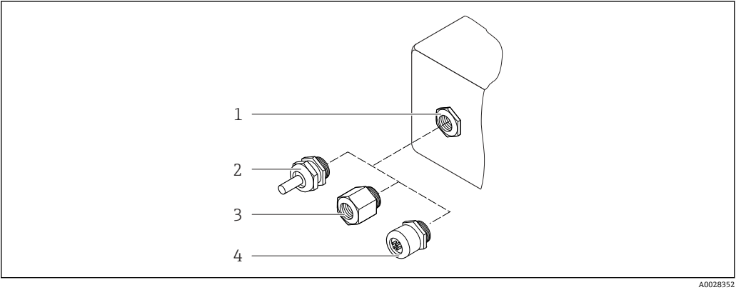
43 允许的电缆入口/缆塞 1 内螺纹 M20 × 1.5 2 缆塞 M20 × 1.5 3 转接头，适用 G ½"或 NPT ½"内螺纹电缆入口 4 设备插头
