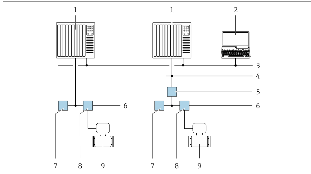
图 48 通过 FOUNDATION Fieldbus 网络进行远程操作
