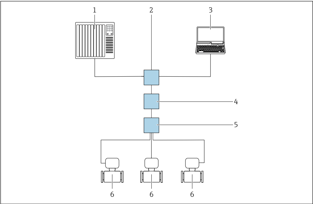
图 56 通过 APL 网络进行远程操作
