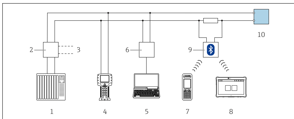
47 通过 HART 通信进行远程操作（无源信号）
