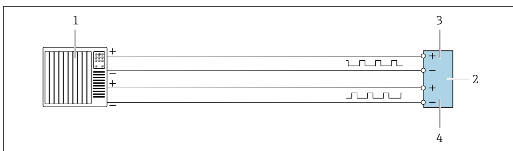
図 22 ダブルパルス出力（アクティブ）の接続例
