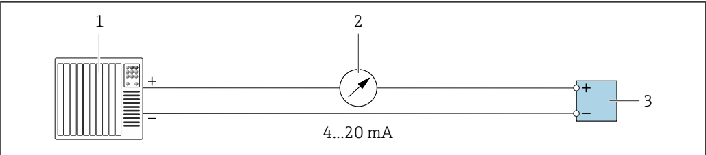
18 4～20 mA 電流出力（アクティブ）の接続例
