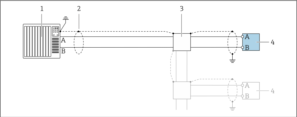
17 Modbus RS485（非危険場所および Zone 2; Class I, Division 2 用）の接続例
