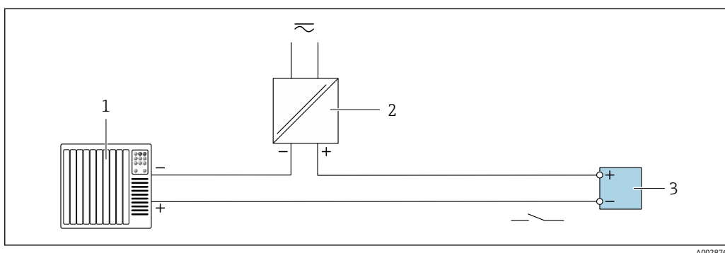
図 21 スイッチ出力（パッシブ）の接続例
